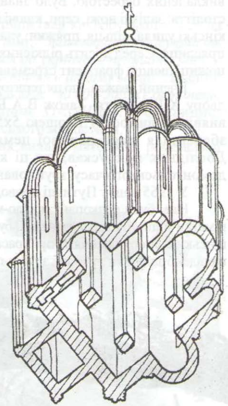
Реконструкція (за Г.Н.Логвіним) та оксонометрія (за Г.К.Вагнером) путивльського храму
