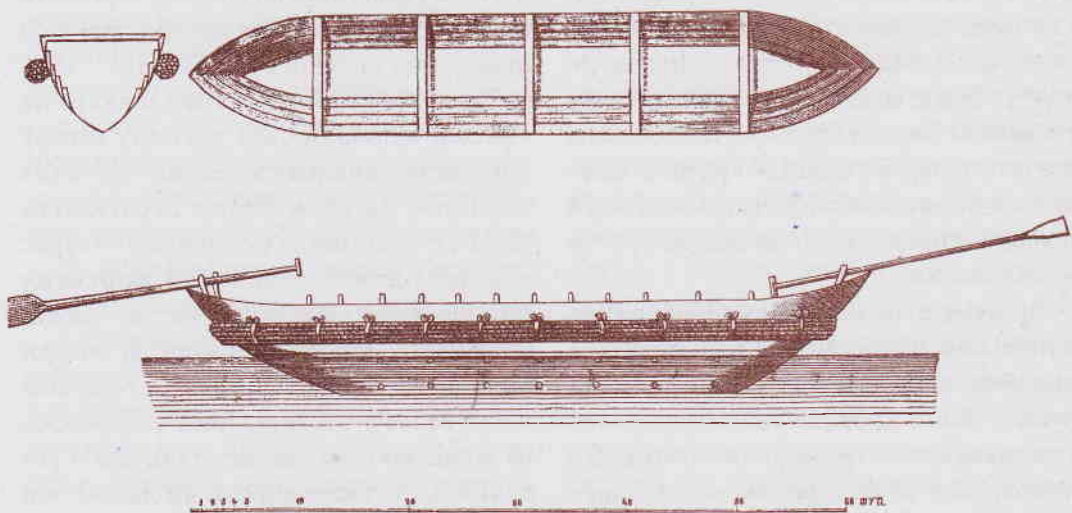
Схема козацької чайки за Г. де Бопланом
