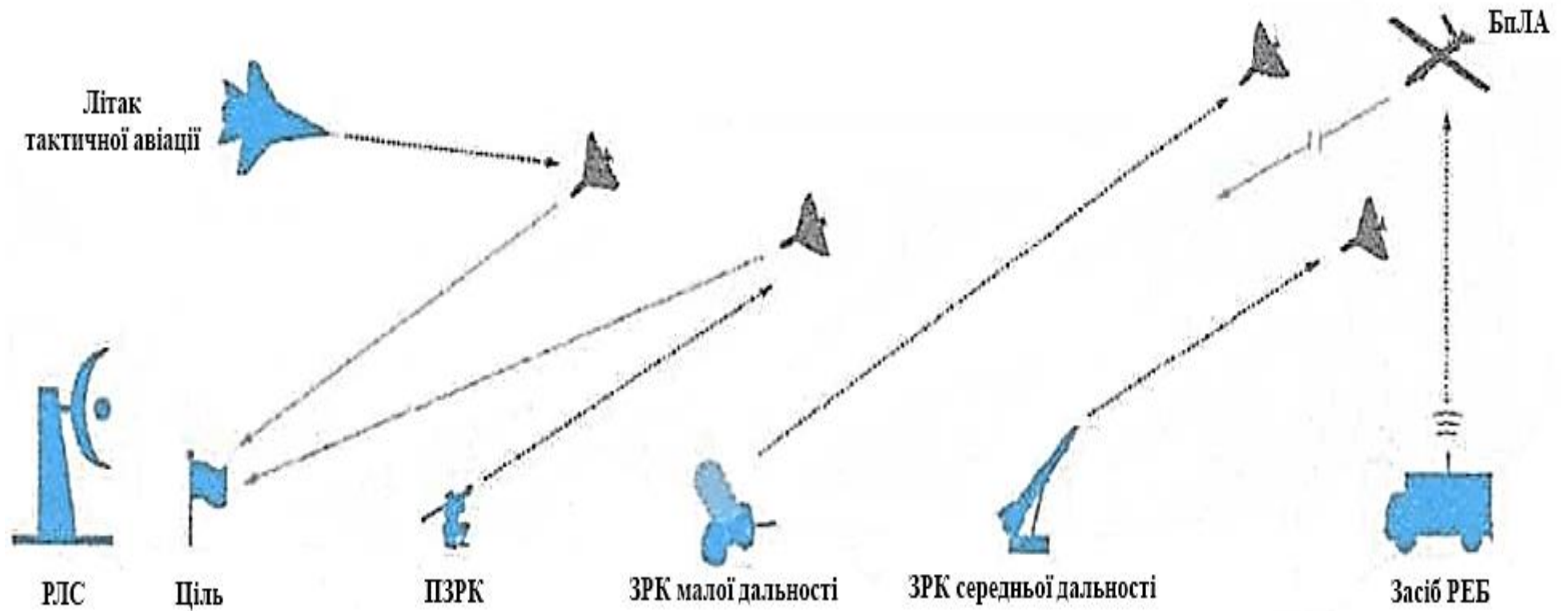
Рисунок 1.7 – Система боротьби з БпЛА типу дронів-камікадзе
