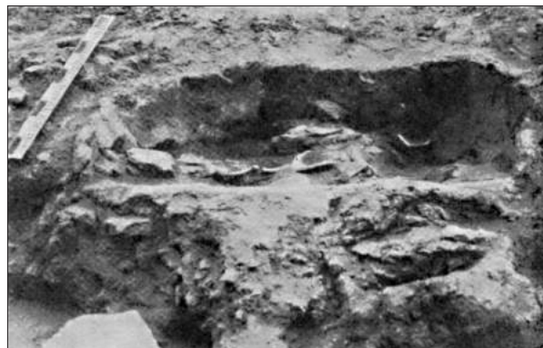
Жванець-Щовб. Гончарна піч, завантажена посудом.
