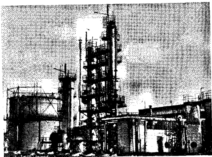
Діюча установка інертного газу Кременчуцького нафтопереробного заводу.
