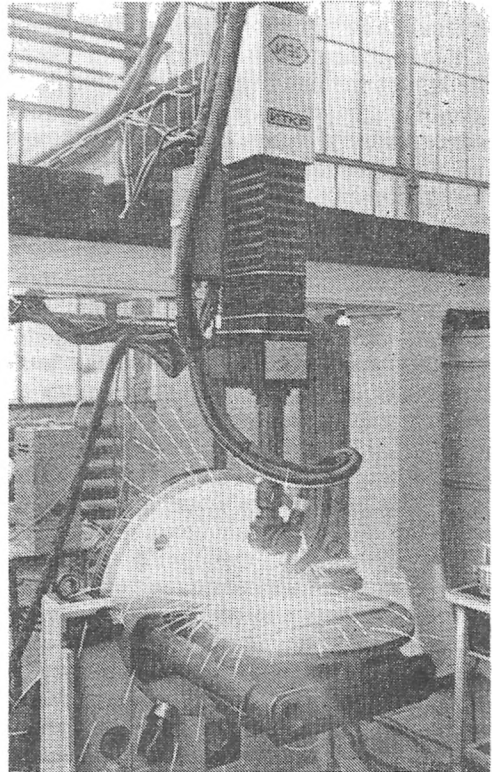
Відзначений золотою медаллю осінньої ярмарки 1980 р. в м. Пловдиві промисловий робот для дугової зварки, що працює на заводі «Ленінська кузня». 1981 р.
