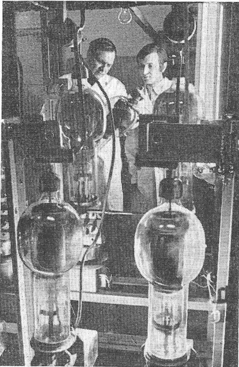
Монтаж ізохронного цилотрона «У-240» в Інституті ядерних досліджень АН УРСР. 1976 р.
