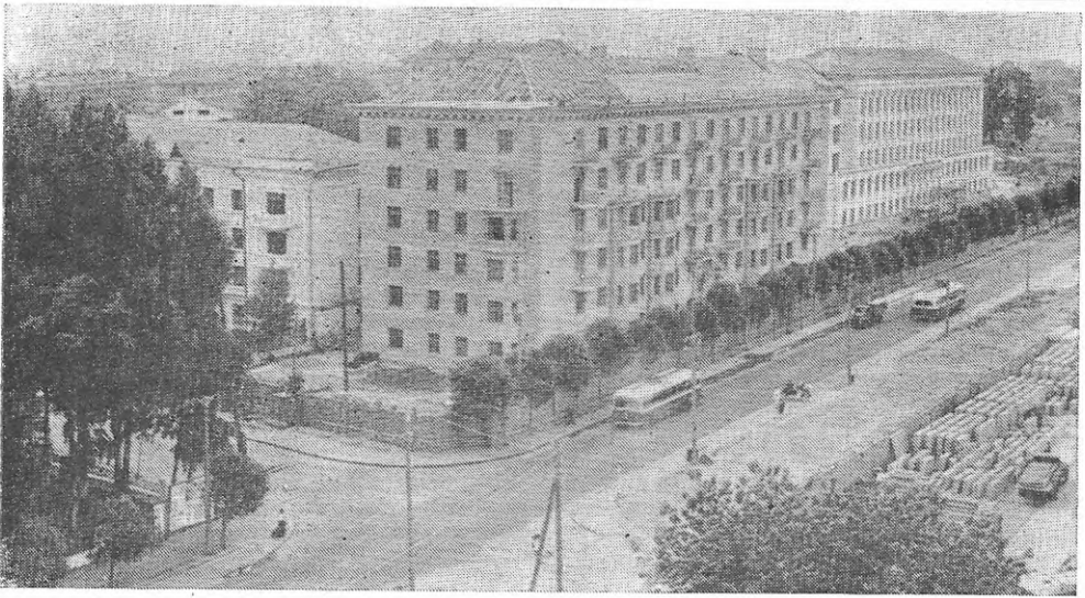
Будівництво житлових будинків по Повітрофлотському проспекту. 1956 р.
