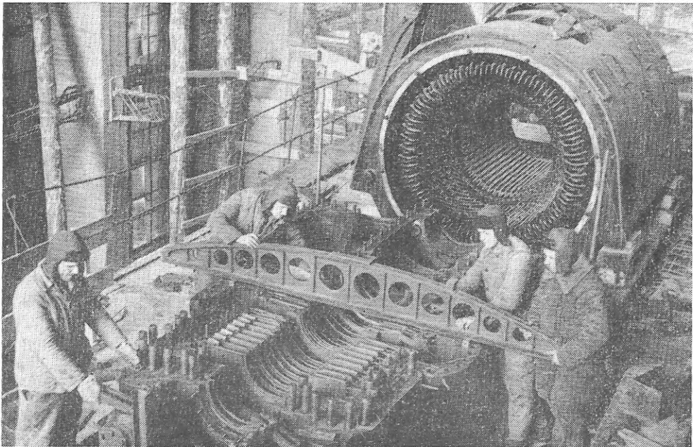
Монтаж турбогенератора на Київській теплоелектроцентралі. 1945 р.
