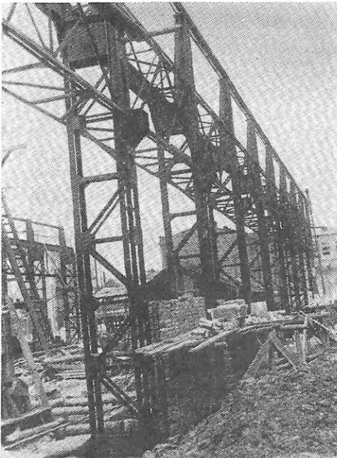
На будівництві ковальського цеху заводу «Ленінська кузня». 1932 р.
