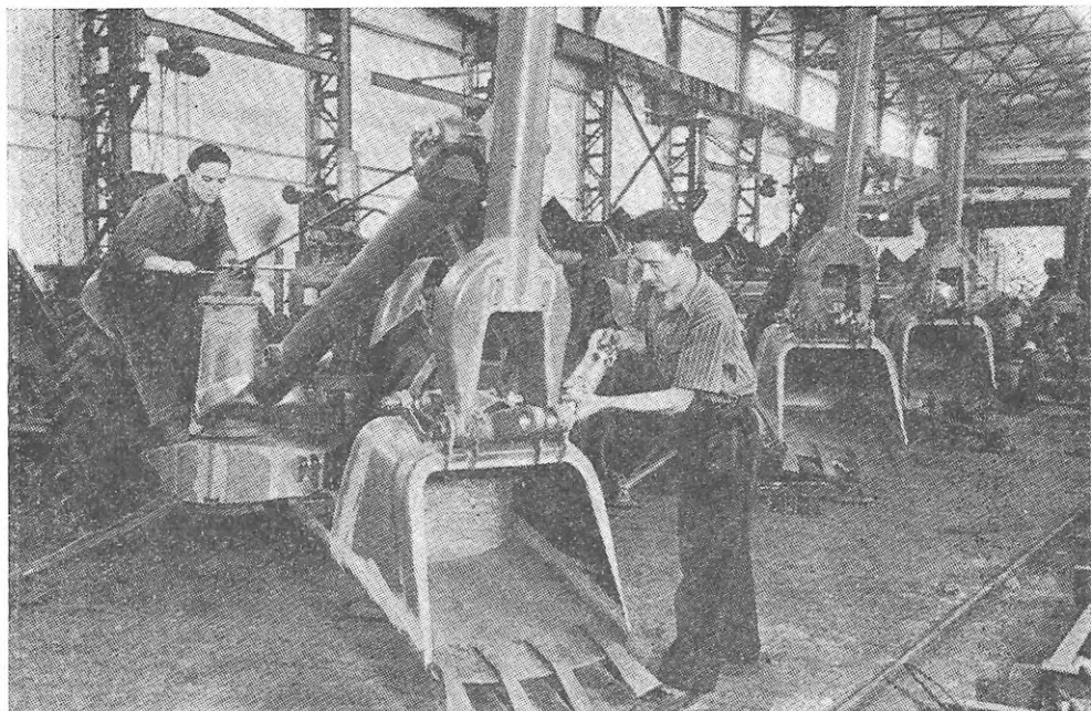
Складання нових універсальних екскаваторів на заводі «Червоний екскаватор». 1955 р.
