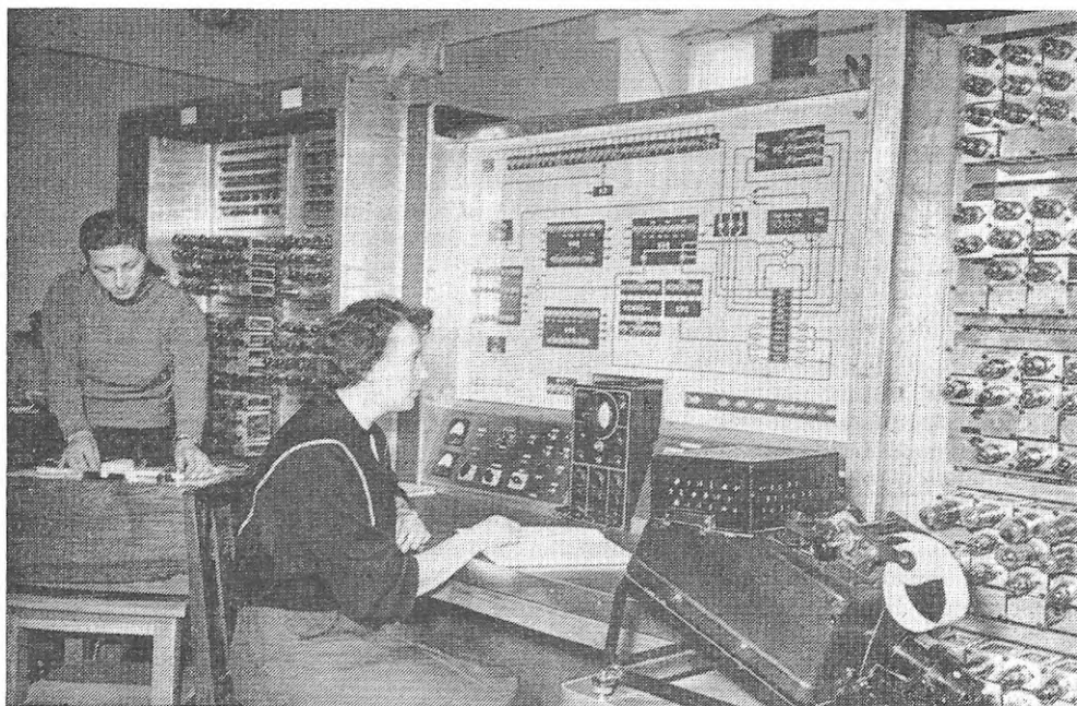
Перша в СРСР і Європі спеціалізована цифрова електронно-обчислювальна машина «СЭОМ» у Обчислювальному центрі АН УРСР. 1958 р.
