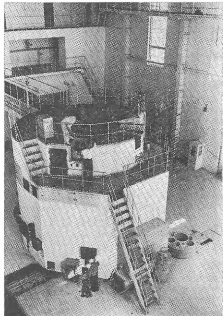
Атомний реактор Інституту фізики АН УРСР. 1960 р.
