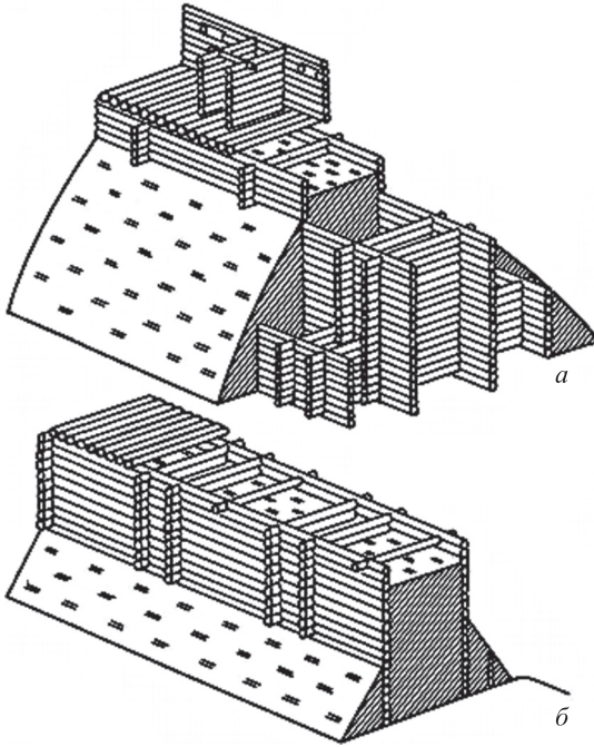
Рис. 1 Реконструкція валу за М. Кучерою, зруб-на конструкція (а – з заборолами; б – без заборол)
