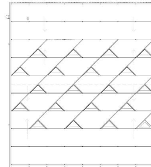
План перекрытия со световыми фонарями
