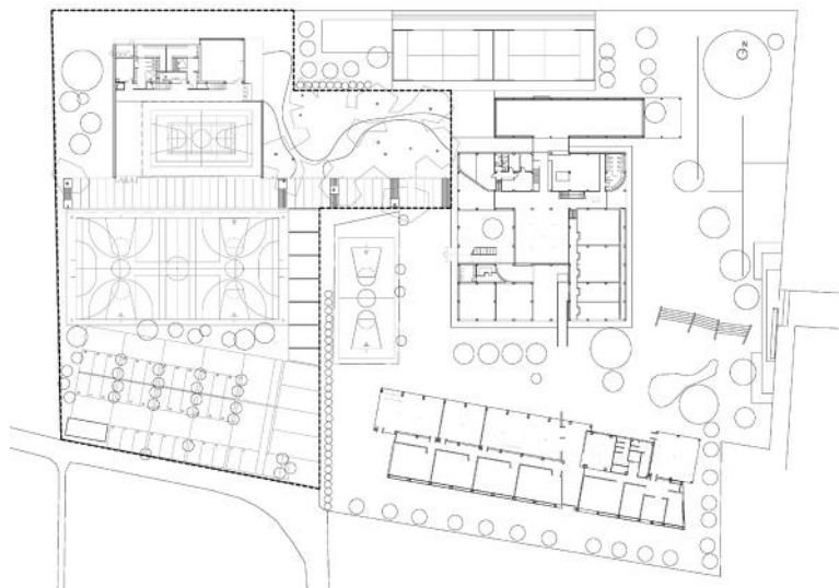
Генплан школы
