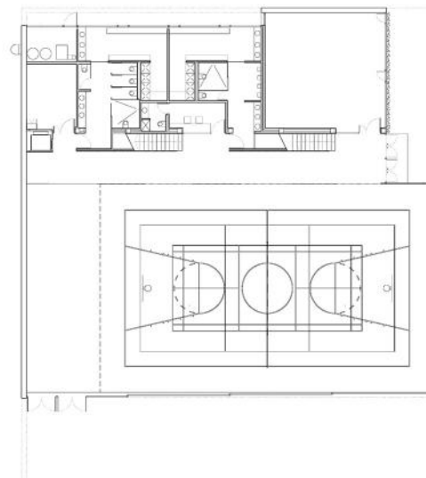
План учебного зала
