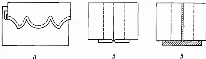
Рис. 1. Вистрочний шов.
