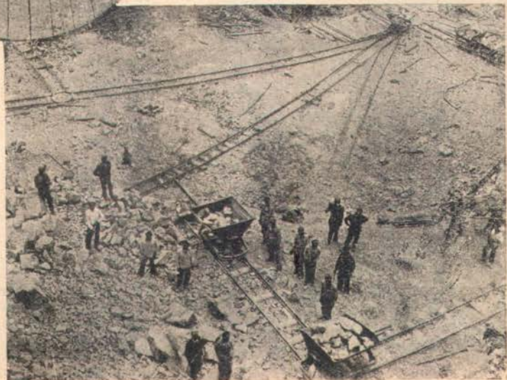
Добутий на кар'єрі граніт вантажать на вагонетки
