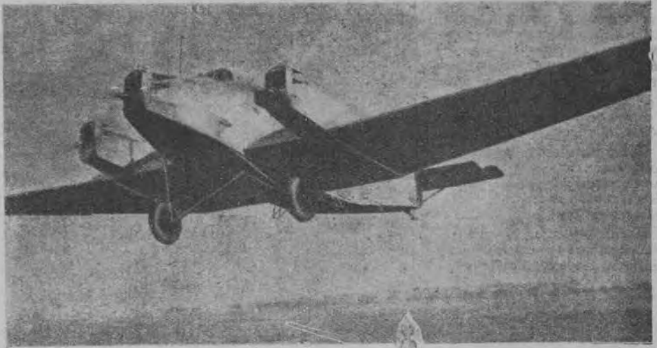
„Юнкерс G 31“—останній аероплан цієї фірми. Розмах крил понад 30 метрів, поверхня понад 100 кв. метрів, спільна потужність трьох моторів—1000 кінських сил
