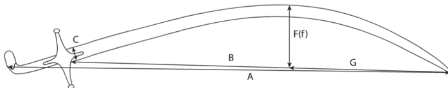
Рис. 2. А – Загальна довжина; В – довжина клинка; С – ширина клинка біля п'яти; F – кривина клинка, або перпендикуляр, опущений від найвищої частини леза (поряд у дужках – від обуха) до відрізка, проведеного між вістря клинка і п'ятою; G – довжина відрізка од вістря до опущеного перпендикуляра, точка або зона найбільшої кривини
