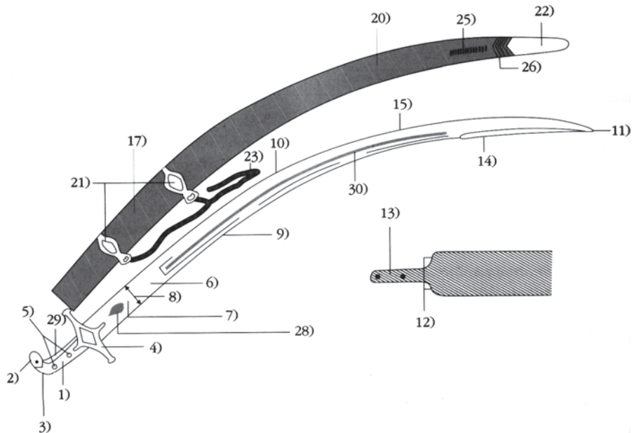
Рис. 1. 1) Daste, Qabze, Moshte [Руків'я]; 2) Sar daste, Kula, Kolah [Верхів'я]; 3) Tahe shamshir [Кантурець]; 4) Volchaq, Sibil [Кільйон]; 5) Mileye etesal, Mikh-e daste [Нюму]; 6) Tigheye [Клинок]; 7) Vadane [Штаба]; 8) Pahna [Ширина клинка]; 9) Labeye posht [Обух і спинка клинка]; 10) Labeye ru [Лезо]; 11) Nish, Nok, Sare tigh [Вістря]; 12) Kalf [П'ята й плічки]; 13) Ut-i-shamshir [Хвостовик]; 14) Pakh [Єлмань]; 15) Mahal zadan zarbe [„Центр вібрації” – ділянка клинка, на якій шабля розвиває найвище січне зусилля; не збігається з точкою рівноваги!]; 16) Jazohar-e tigh [Структура або матеріал клинка]; 17) Ghalaf [Піхви]; 18) Zag-e sefid [Речовина для монтажу ефеса з клинком]; 19) Qabze [Щічки руків'я – іноді руків'я]; 20) Saghri, Saghari [Шагренева шкіра на піхвах]; 21) Varband, Baste ghalaf [Обіймиці]; 22) Tah-e Ghalaf [Наконечник]; 23) Band-e shamshir, Namayel [Паски або португезя]; 24) Shamshir gardan [Піхви разом з пасками]; 25) Simduzi [Повздожний дротяний шов на піхвах]; 26) Ristanbafi [Шиття при кінці піхов, зазвичай нитками двох різних кольорів]; 27) Tazinat [Орнаментация клинка]; 28) Toranj [Картуш]; 29) Ahanak [Низ кантурія]; 30) Nav [Доли]
