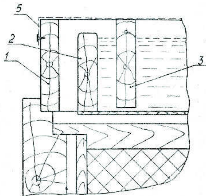
Рис. 2. Конструкція годівниці: 1 — каркас-обв'язка; 2 — роздільна дощечка 220×60; 3 — роздільна дощечка з пазом 220×70; 4 — дно з ДВП 250×470; 5 — плівка поліетиленова.
