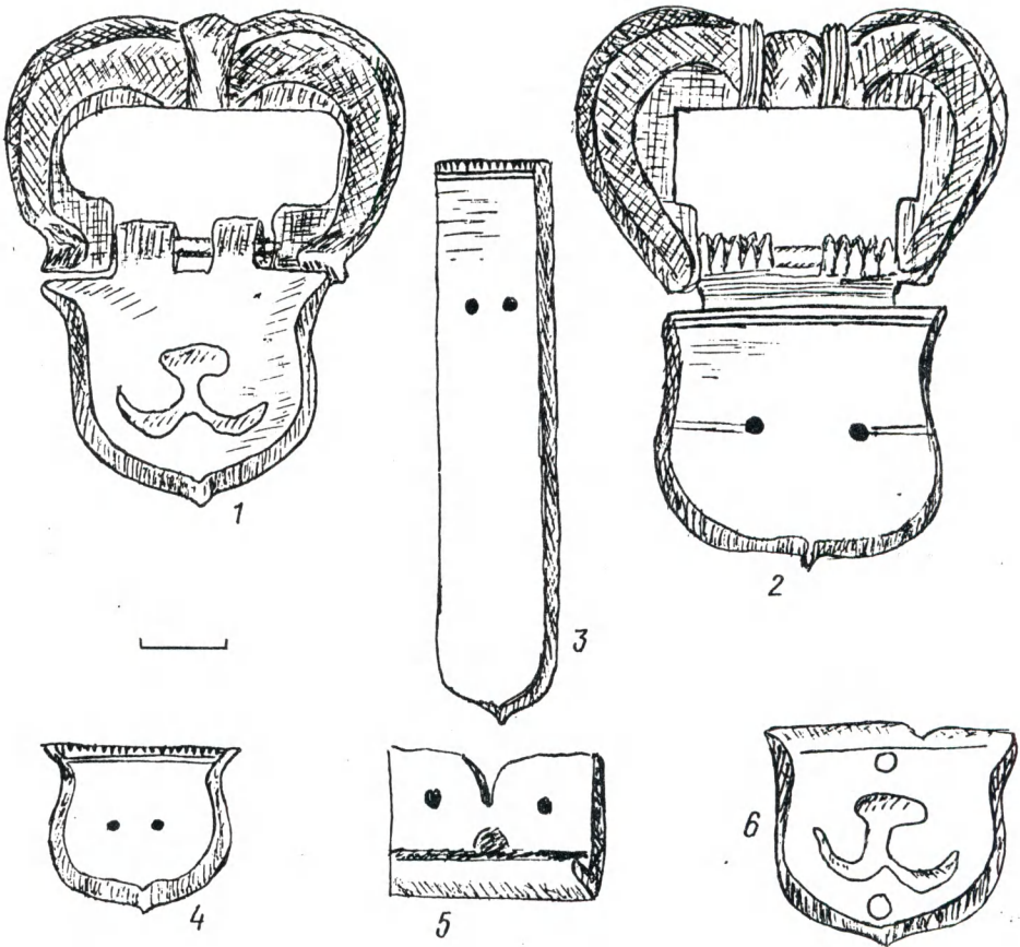
Рис. 11. Предметы поясных наборов.
