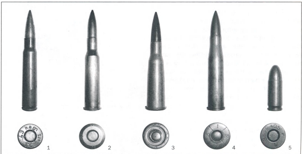
Таблиця 2. Зразки набойів та клейм на деннях гільз стрілецької зброї:
