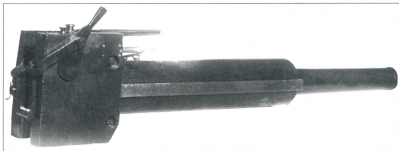
Танкова гармата Л-10: нею була оснащена частина танків 8-ї танкової дивізії
