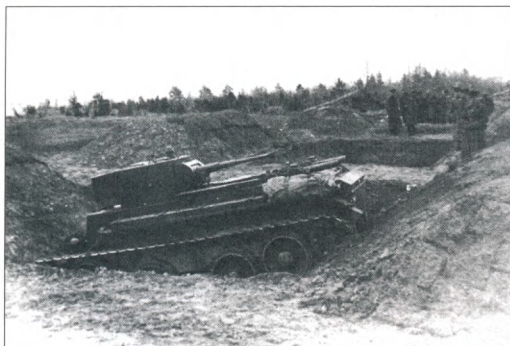
Випробування танка на полігоні: BT-7 долає протитанковий рів
