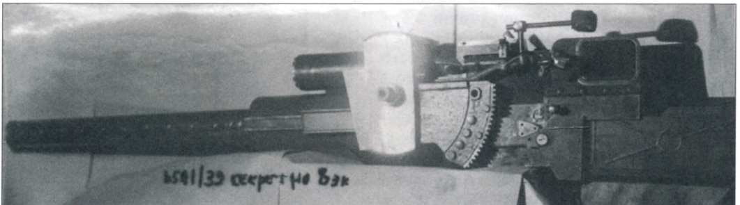
Танкова гармата Л-11: цією артсистемою були укомплектовані всі Т-34 і КВ-1 8-ї танкової дивізії. Тут і далі — фото з фондів РГВА, надав Ю. Пашолок, публікуються вперше
