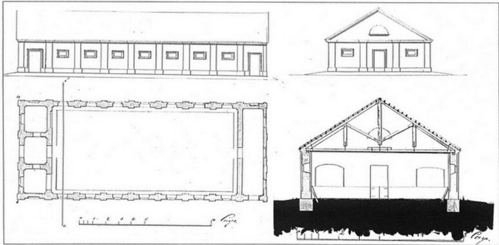
Рис. 30 План кам'яного манежу в с. Привольне Новоросійського (Херсонського) військового поселення кавалерії (1854) *
