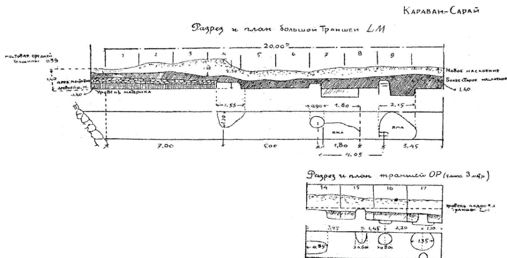
Рис. 4. Планы и разрезы двух траншей, заложенных археологической экспедицией Крымсовнаркома, Крымцика и Научной ассоциации востоковедения Союза ССР в 1925г. на территории каравансарая в Старом Крыму. Рисунок П. И. Голландского [11, с. 18].
