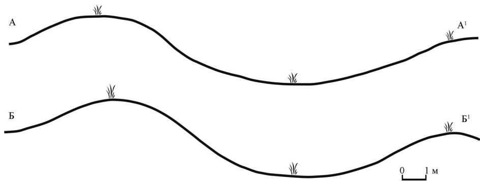
Рис. 4. Профили валов и рвов цитадели Гороховатского городища
