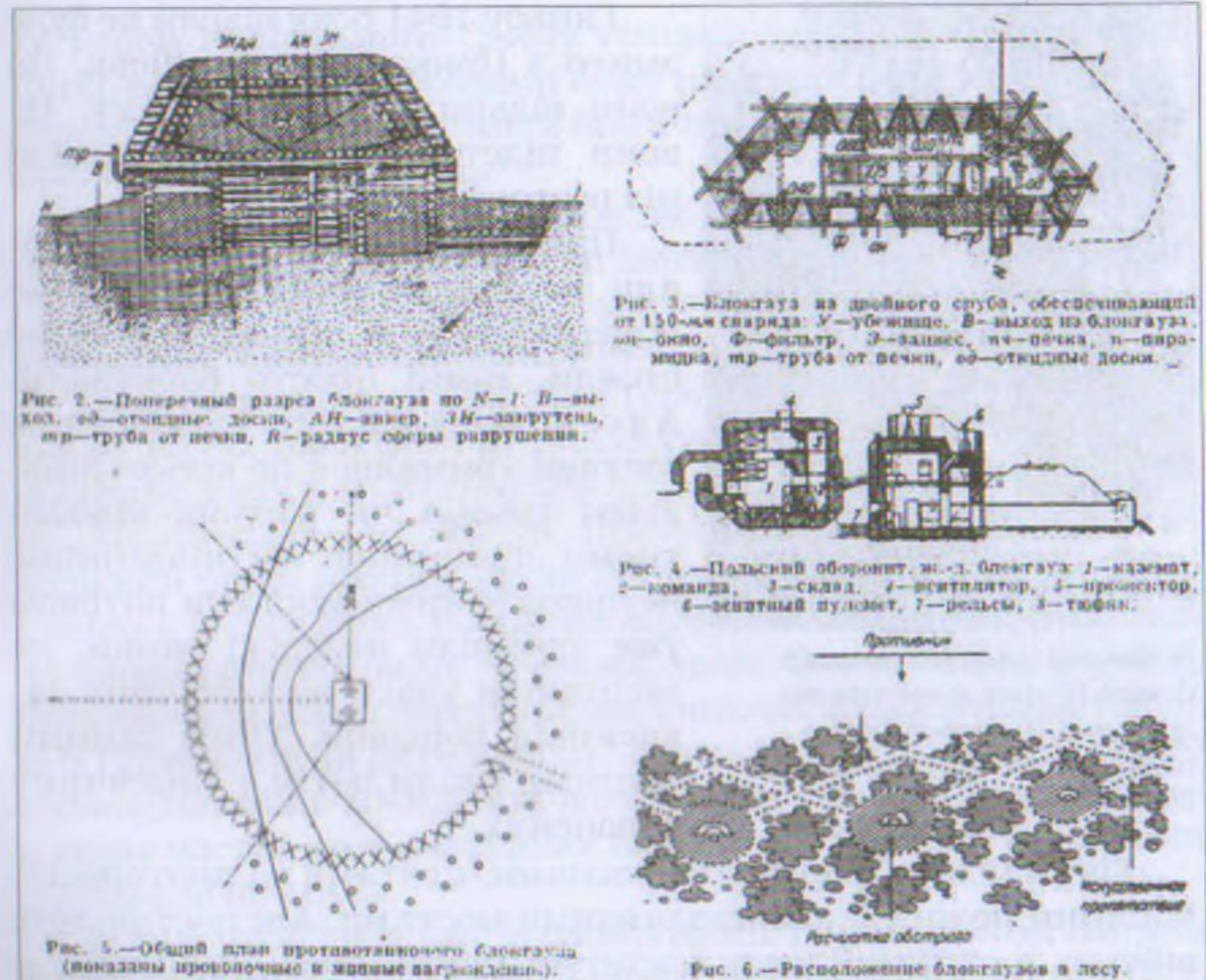
Блокгауз. З Радянської військової енциклопедії 1932–1933 рр.
