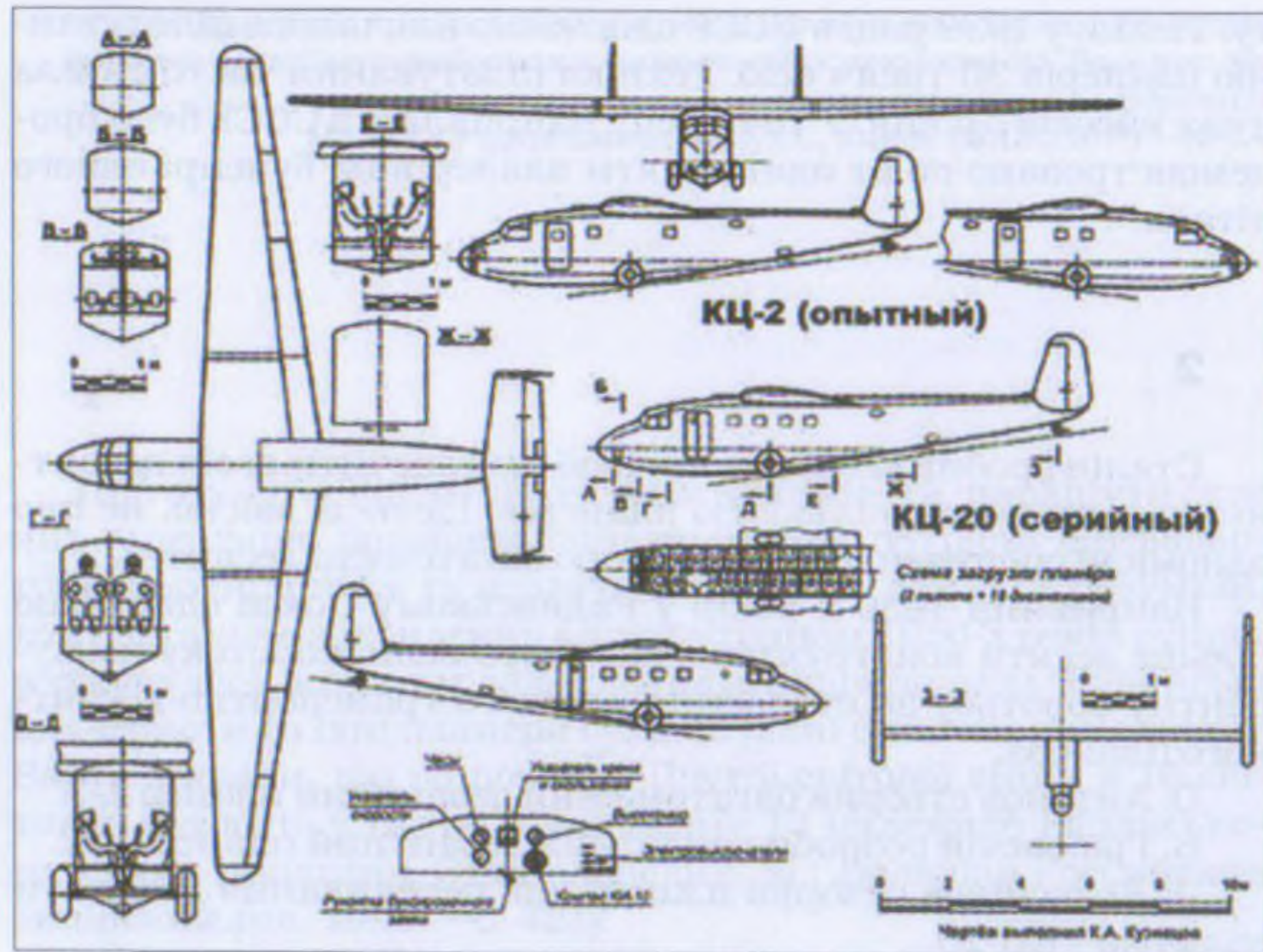
Планер КЦ-20. Креслення
