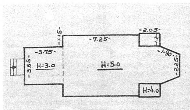
Рис. 3. Івано-Богословська церква в с. Бармаки, 1773 р. Схема плану, 1959 р. [9, арк. 66].
