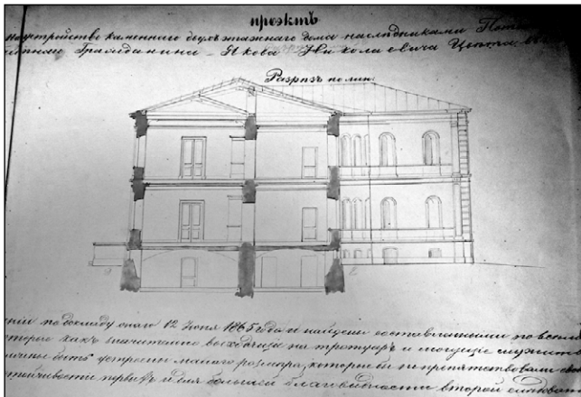
Розріз будівлі.
