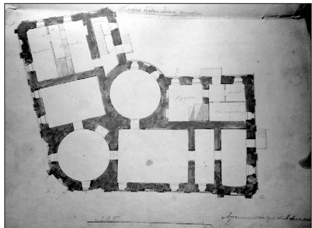
План підвального поверху.
