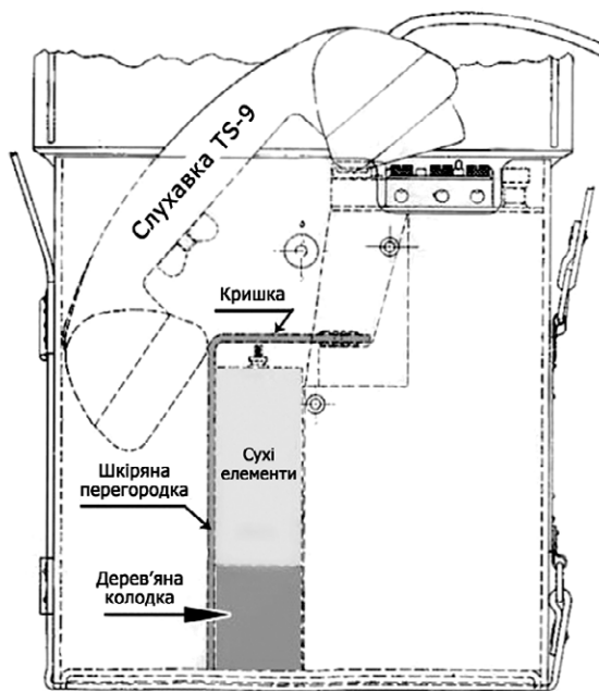
Рис. 3. Схема розміщення додаткових сухих елементів живлення в апаратах ЕЕ-8, які надходили до СРСР по лінії Амторгу.
