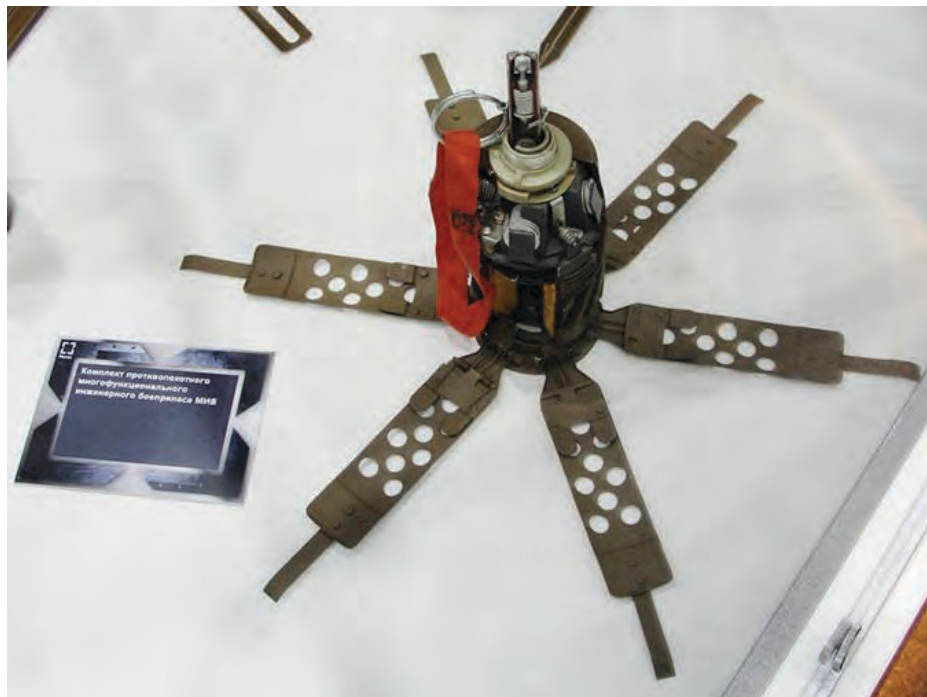
Малюнок 6.10.3 – Міна-граната МІБ, в бойовому положенні
