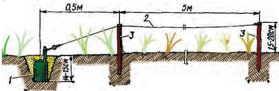
Малюнок 6.3.3 – Встановлення міни ОЗМ-3 в ґрунт: 1 – міна; 2 – дротова розтяжка; 3 – кілочка розтяжки
