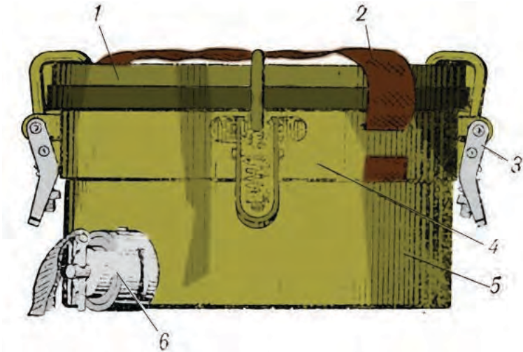
Малюнок 8.6.1 – Міна МЛ-1: 1 – протищуповий датчик; 2 – ручка із тасьми; 3 – замок; 4 – кільце; 5 – блок управління; 6 – пусковий механізм
