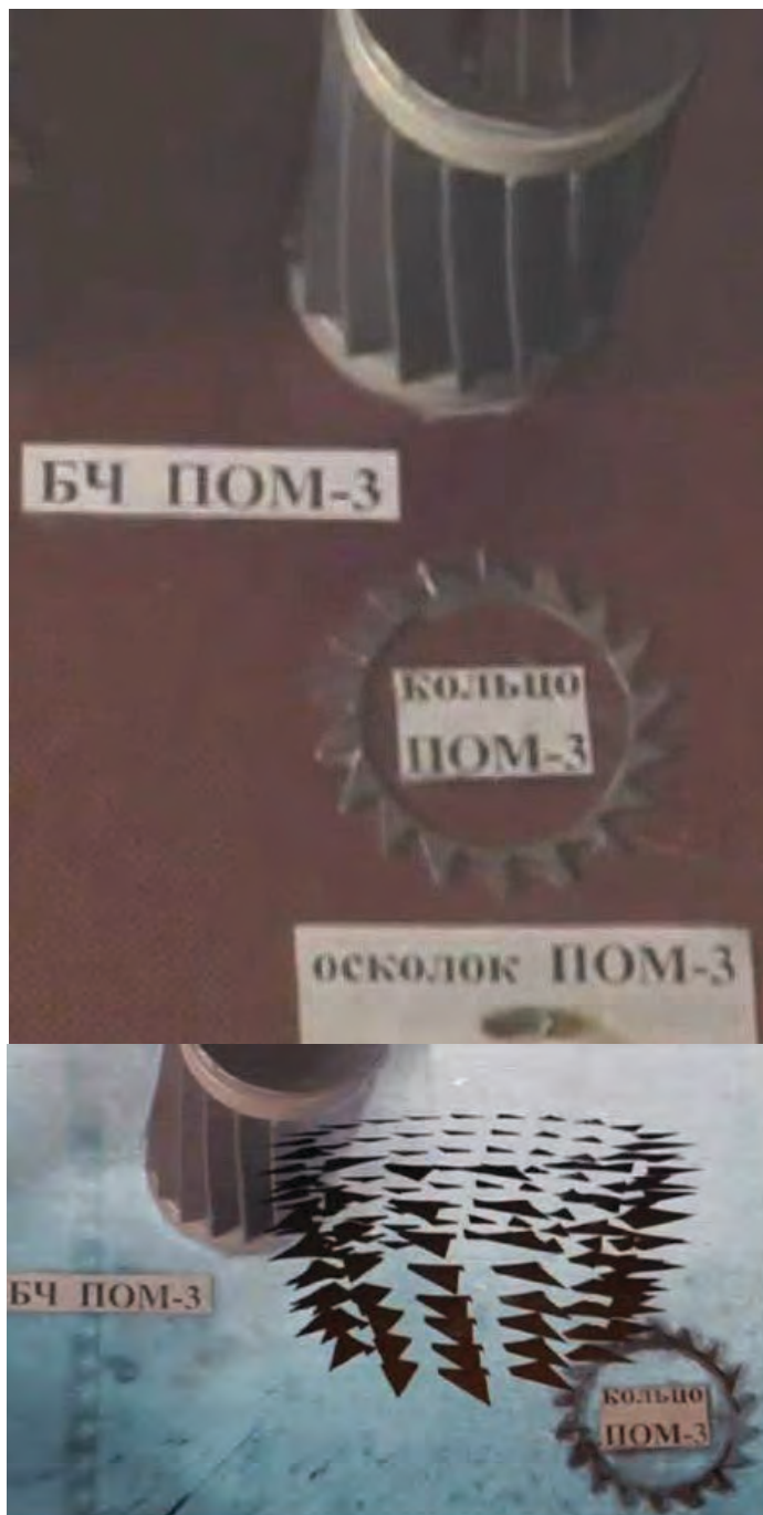
Малюнок 7.8.4 – Бойова частина міни ПОМ-3
