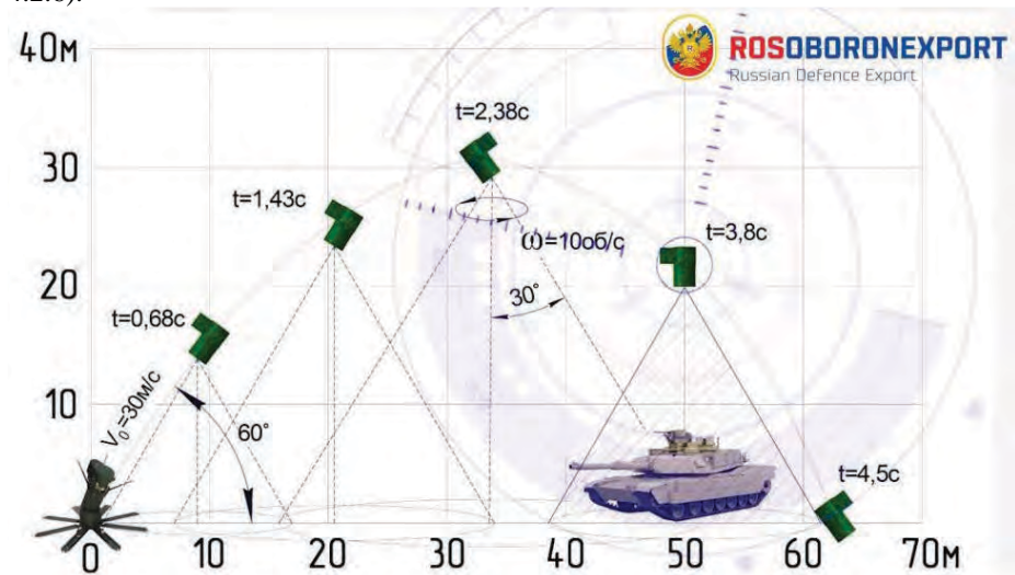
Малюнок 4.2.4 – Схема принципу роботи міни ПТКМ-1Р
