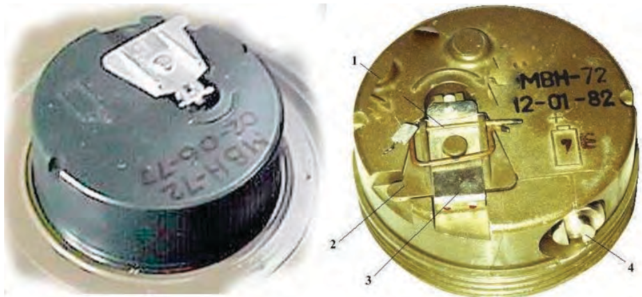
Малюнок 1.4.10 – Детонатор МВН-72. Цифрами зазначено: 1 – штилька; 2 – відкидна кришка годинникового механізму; 3 – запобіжна чека; 4 – пробка гнізда джерела струму
