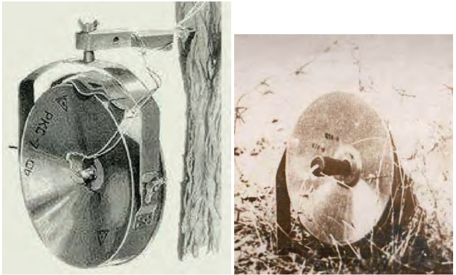
Малюнок 7.5.2 – Міна МОН-100, Варіанти встановлень: зліва – на дерево; справа – на ґрунт
