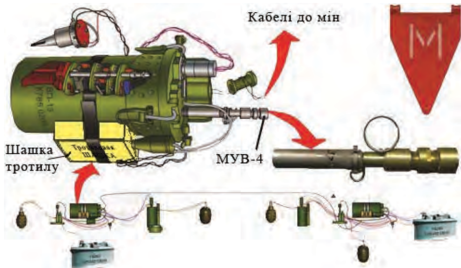
Малюнок 7.10.8 – ВБУ-П з тротиловою шашкою. Знизу показано варіант встановлення ВБУ-П з гранатами Ф-1 та РГД-5, в якості мін – в них замість запалів вставлено електродетонатори. Зверху справа – знак «Міни»
