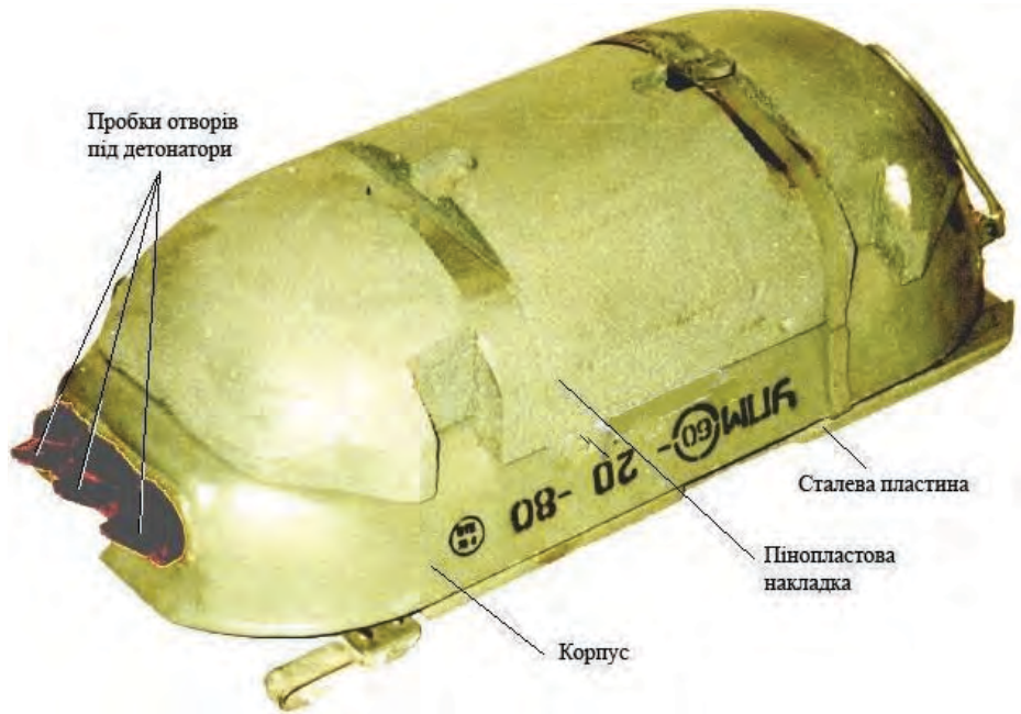
Малюнок 9.6.1 – Міна УПМ, загальний вигляд
