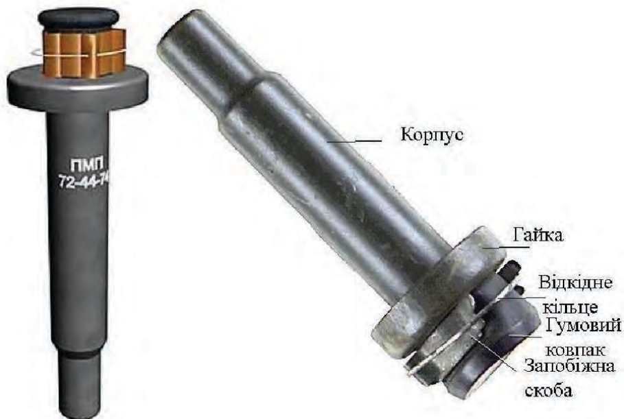
Малюнок 5.7.1 – Міна ПМП, загальний вигляд та деталі будови
