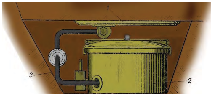
Малюнок 8.4.2 – Встановлення міни МС-6Щ: 1 – протищуповий датчик; 2 – блок управління; 3 – з'єднувальний кабель
