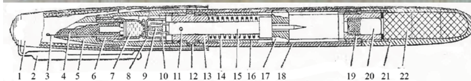
Малюнок 8.10.4 – Детонатор МВ-3, Загальний вигляд, в розібраному стані та в розрізі: 1 – кришка; 2 – утримувач; 3 – перо; 4 – вкладиш; 5 – наконечник; 6, 13, 19 – втулки; 7 – піпетка для чорнила; 8 – ковпачок; 9 – металоелемент; 10 – різак; 11 – чека; 12 – кільце; 14 – бойова пружина; 15 – ударник; 16 – корпус; 17 – запобіжна гайка; 18 – зовнішня трубка; 20 – капсуль-детонатор МГ-8-Т; 21 – гільза; 22 – заряд ВР. МВ-1, МВ-2 влаштовані так само
