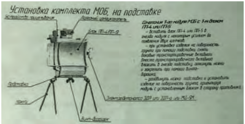
Малюнок 7.7.4 – Установка МОБ на подставці (з інструкції з експлуатації АО НІІІІ та МО РФ); Цей варіант використовується при установці міни з натяжним дротом, для кращого маскування
