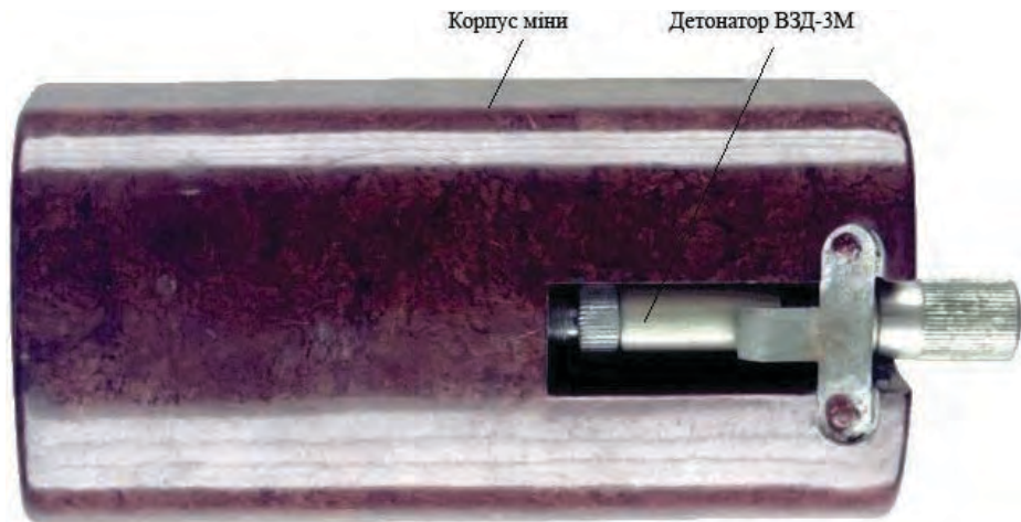
Малюнок 9.3.1 – Міна МПМ, загальний вигляд
