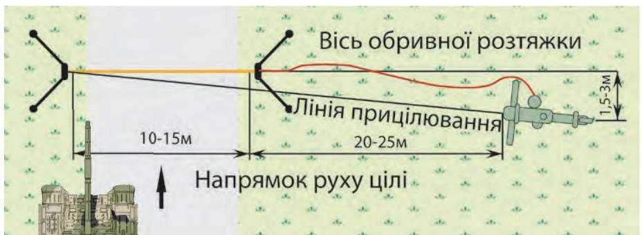
Малюнок 3.1.3 – Схема встановлення міни ТМ-73
