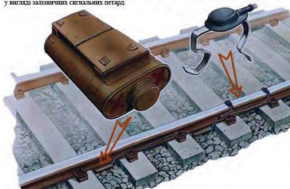
Малюнок 13.4.3 – Петарда в якості детонатора протитранспортної міни
