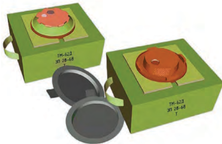
Малюнок 1.10.1 – Міна ТМ-62Д. Зверху – з детонатором МВЧ-62; Знизу – зліва – з детонатором МВЧ-62; Знизу справа – з детонатором МВ-62; Сірого кольору – гумові заглушки гнізд детонаторів
