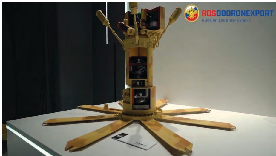
Малюнок 4.2.2 – Розріз міни ПТКМ-Р з рособоронекспорту рф
