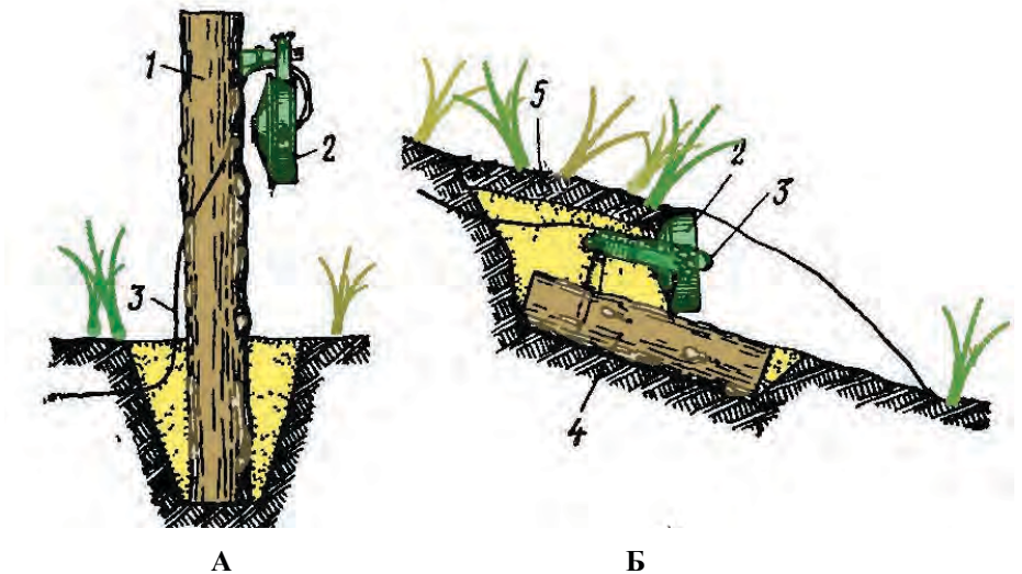
Малюнок 7.5.3 – Схема встановлювань міни МОН-100: А – на стовбурі (дереві); Б – в ґрунті на схилі місцевості з маскуванню під купину; 1 – стовбур; 2 – міна; 3 – електрокабель; 4 – колода, звкопана в ґрунт; 5 – маскуванню дереном
