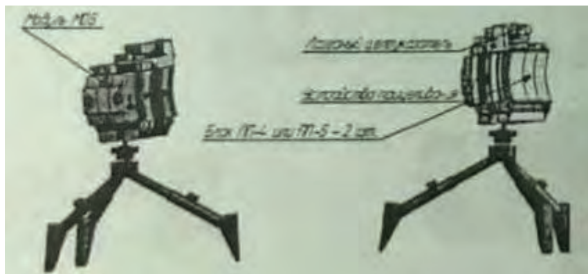
Малюнок 7.7.3 – Установка МОБ на тренозі з двома модулями, встановленими в тандем (з інструкції з експлуатації АО НІІІІ та МО РФ); Кількість ГЗЕ зростає вдвічі
