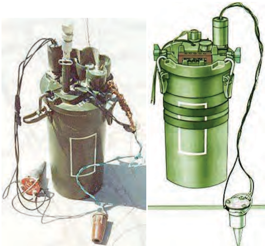
Малюнок 7.10.1 – Підриваючий пристрій НВУ-П, загальний вигляд – зліва, та підготовлений для перевірки працездатності з сейсмотатчиком
