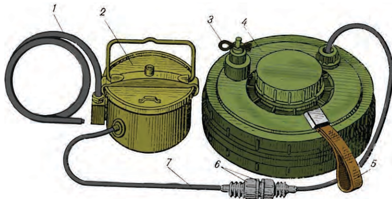
Малюнок 8.5.1 – Міна МС-6М: 1 – пусковий трос; 2 – блок управління; 3 – чека вмикача; 4 – протиміношукачевий датчик; 5 – ручка; 6 – напівмуфта; 7 – кабель
