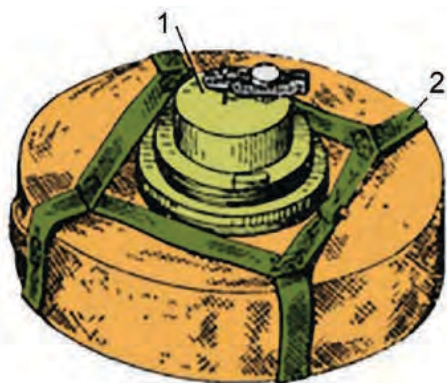
Малюнок 1.8.1 – Зліва: міна ТМ-62Т з детонатором МВП-62 (1) та з'ємною синтетичною ручкою (2); Справа: міна ТМ-62Т з детонатором МВ-62 та нез'ємною ручкою
