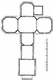
План Миколаївської церкви в с. Синяві Васильківського повіту Київської губернії. Опубліковано: Г. Г. Павлуцький. Дерев'яні і кам'яні храми. К.: 1905 р., с. 109
