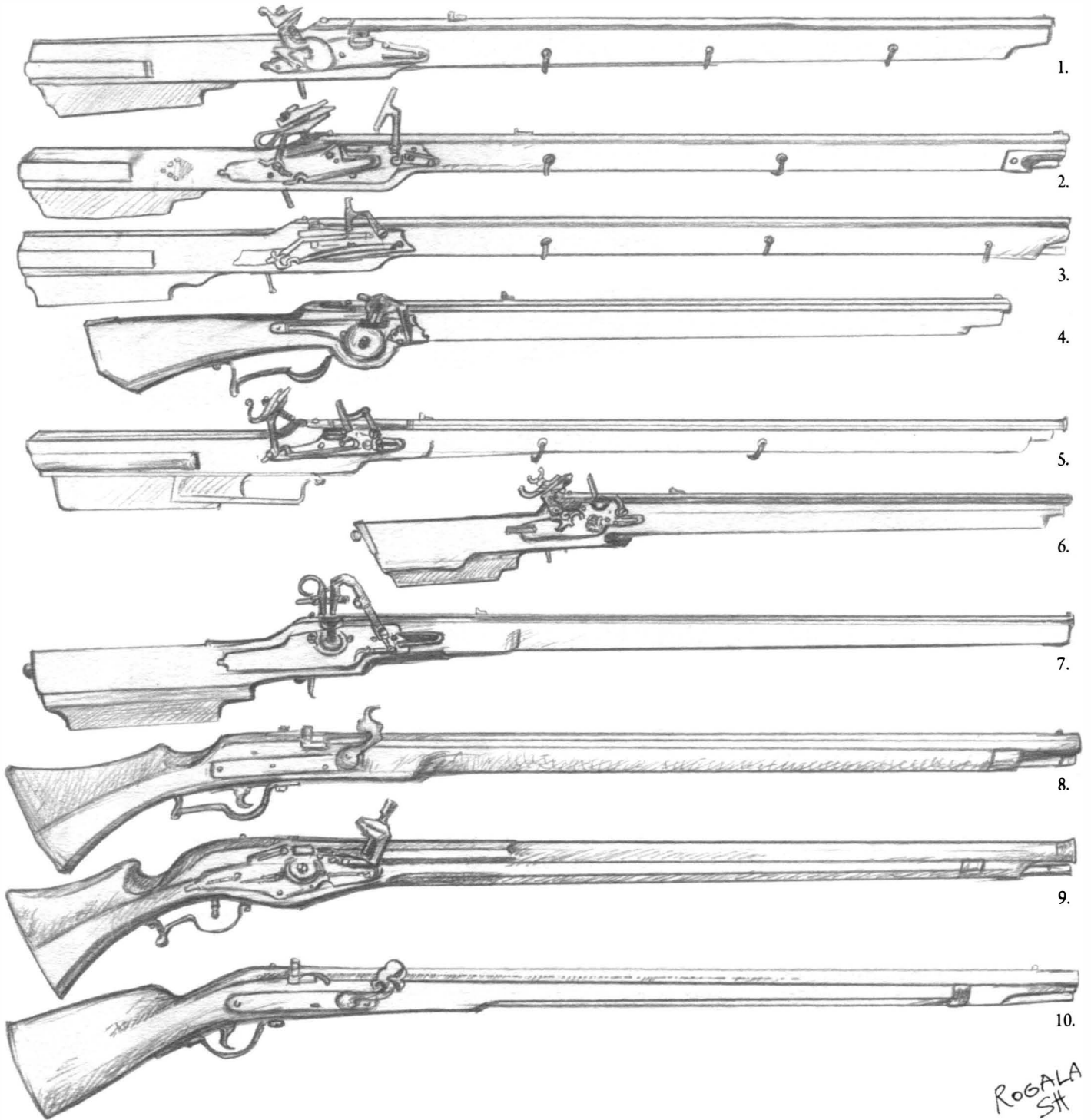
Види козацьких мушкетів. 1. Мушкет із європейським замком, із запобіжником. 2, 3, 5. Мушкети з кременевим московським замком. 4, 6. Кавалерійські бандолети. 7. Мушкет із коліщатим замком (1–7. За знахідками під Берестечком). 8. Гнотовий мушкет європейського зразка. 9. Коліщатий мушкет європейського зразка, перша чверть XVII ст. 10. Гнотовий мушкет 70-х років XVII ст.
