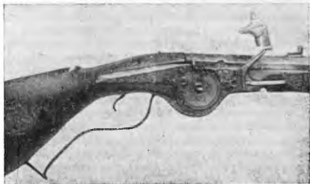
Колесцовый замок ручницы. Первая половина XVII в.
