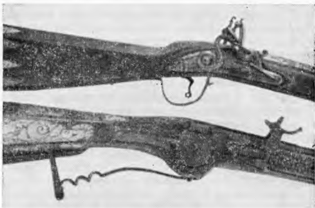
Ударно-кремневый замок ручницы и колесцовый замок аркебуза. Первая половина XVII в.
