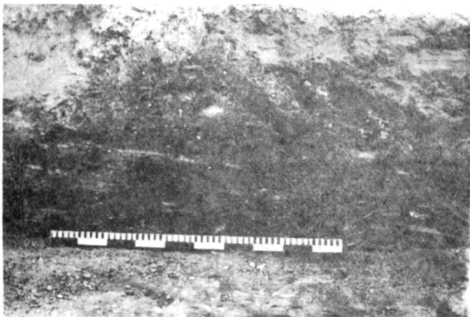
Рис. 2. Розріз валу (ділянка Р-19)
