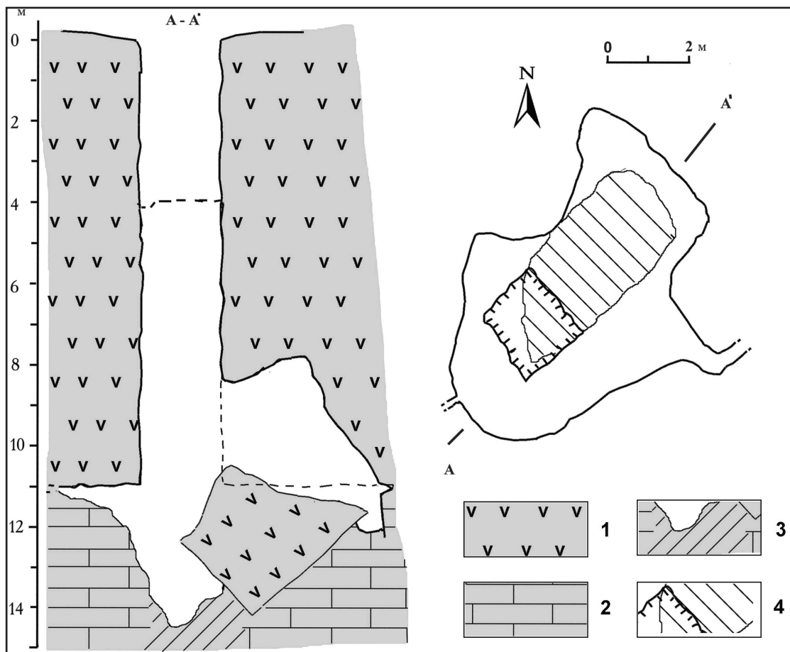
Рис. 1. План і розріз Турецької Крилиці.
