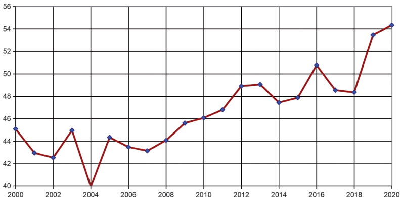
Рис. 25. Динаміка рівня викидів CO 2 від електро- та теплогенеруючих установок упродовж 2000–2020 рр., CO 2 /MДж
