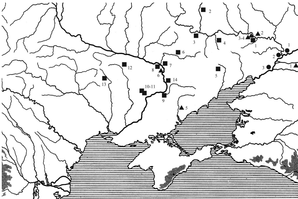
Рис. 5. Карта розповсюдження крем'яних вістрів стріл типів 2 та 4 (частково використано: Кияшко, Поплевко, 2000, Рис. 6) (див. табл. 4). Коло - поселення з вістрями типу 4 (майкопськими): 1 - Костянтинівка; 2 - Самсонівське; 3 - Раздорське I; трикутник - поховання з вістрями типу 4 (майкопськими): 1 - хут. Новий; 2 - Піонерське; 3,4 - Олександрівськ; 5 - Костянтинівка; 6 - о-в Виноградний; квадрат - поховання з вістрями типу 2 (з увігнутою основою): 1 - Олександрівськ; 2 - Олександрія; 3 - Ковалівка; 4 - Радіонівка; 5 - Шахтарськ; 6 - Вербки; 7 - Стара Огринь; 8 - Дніпропетровськ; 9 - Василівка; 10-11 - Кам'янка; 12 - Пісчаний Брід; 13 - Кіровоград; 14 - Кічкас.
