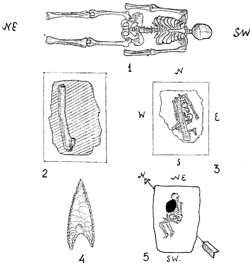
Рис. 4. Кічкас, Дніпрельстан, курган 7: 1 - пох. "Г"; 2 - перекриття пох. "Д"; 3 - пох. "Е"; 4 - крем'яне вістря стріли з пох. "Е"; 5 - пох. "Ж" (за: Смоличев, 1930, рис. 13, 14, 15, 16 та 17).
