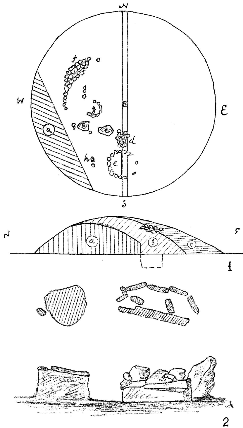
Рис. 2. Кічкас, Дніпрельстан, курган 7: 1 - схематичний план та профіль кургану; 2 - кам'яна гробниця (за: Смоличев, 1930, рис. 6,8 та 7).
