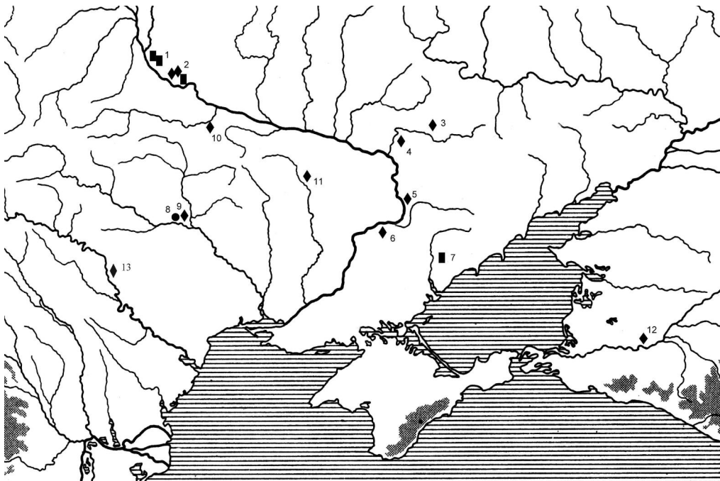
Рис. 1. Карта розповсюдження наверхів кічкаського типу:
