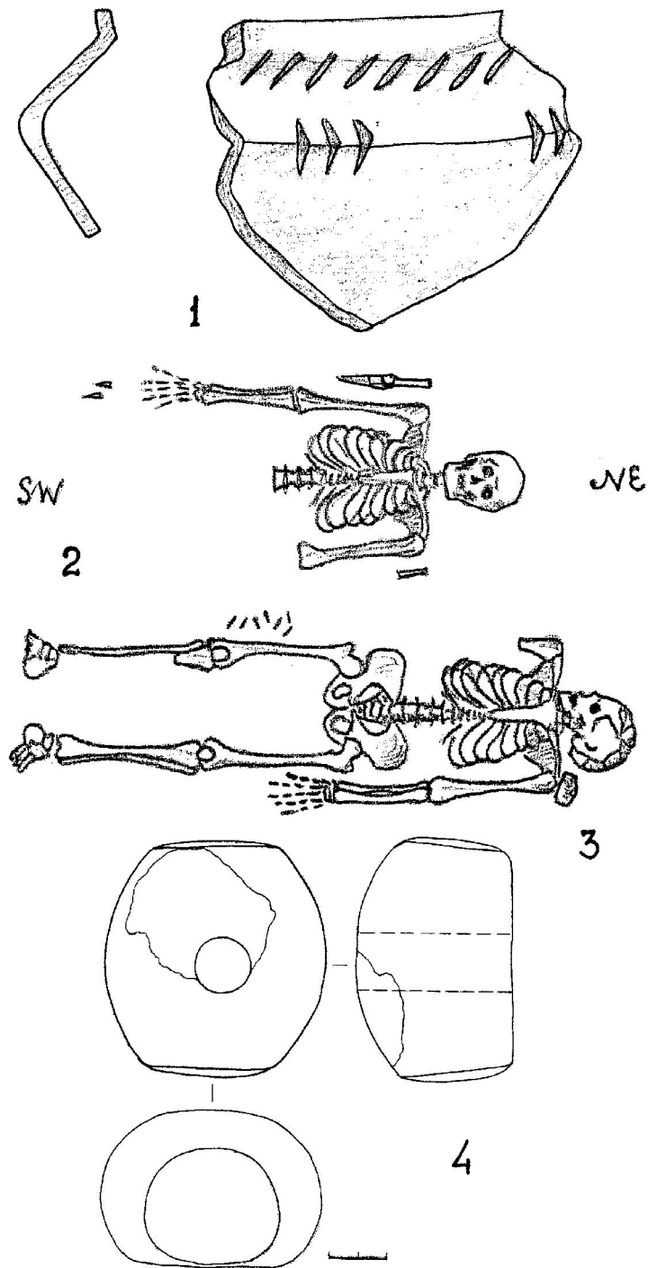
Рис. 3. Кічкас, Дніпрельстан, курган 7: 1 - фрагмент горщика з пох. "А"; 2 - пох. "Б"; 3 - пох. "В"; 4 - кам'яне навершя з пох. "В" (1-3 за Смоличев, 1930, рис. 9,10,11; 4 - рисунок автора).
