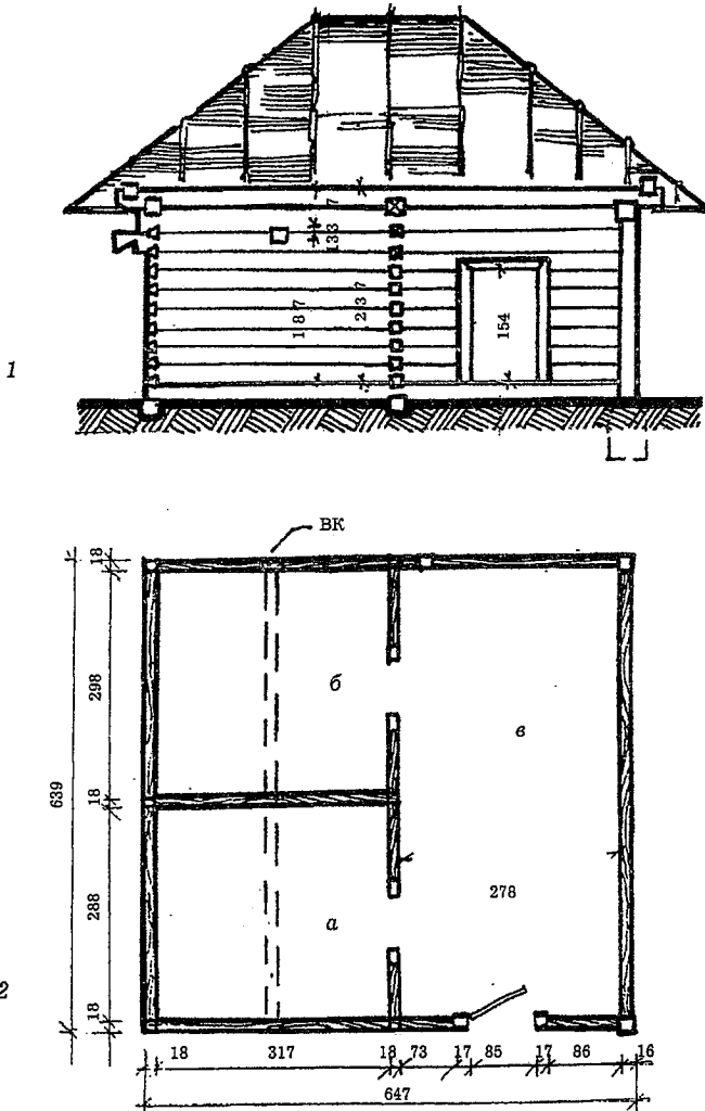
4. „Інбар“ із села Любимівки Вишгородського р-ну Київської обл. Початок ХХ ст.:
