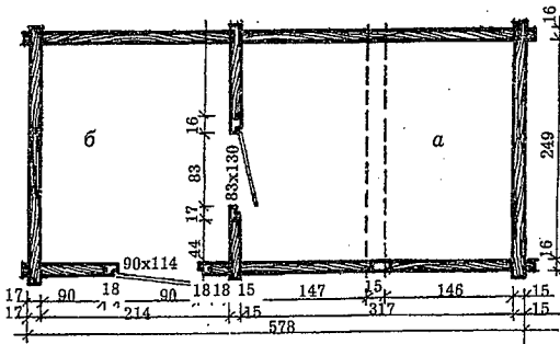
2. Стебка із села Сновидовичів Рокитнівського р-ну Житомирської обл. Середина XIX ст.:
