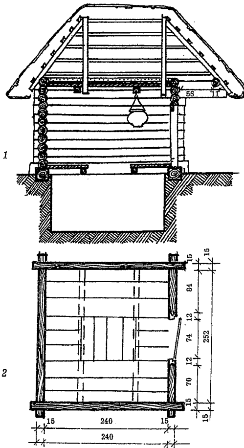
5. Стебка із села Паришева колишнього Чорнобильського р-ну Київської обл. Початок ХХ ст.: 1 — розріз; 2 — план
