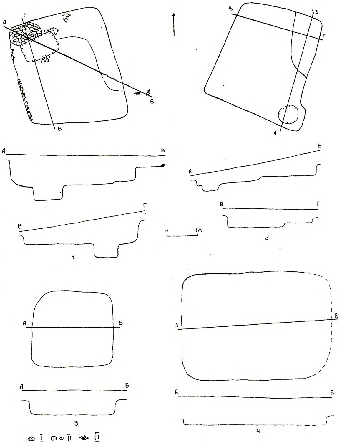
Рис. 11. Пастырське. Плани та перетини ранньосередньовічних напівземлянок № 1 (1), № 3 (2), № 4 (3); № 6 (4), розкопаних у дев'яності роки XX ст.
