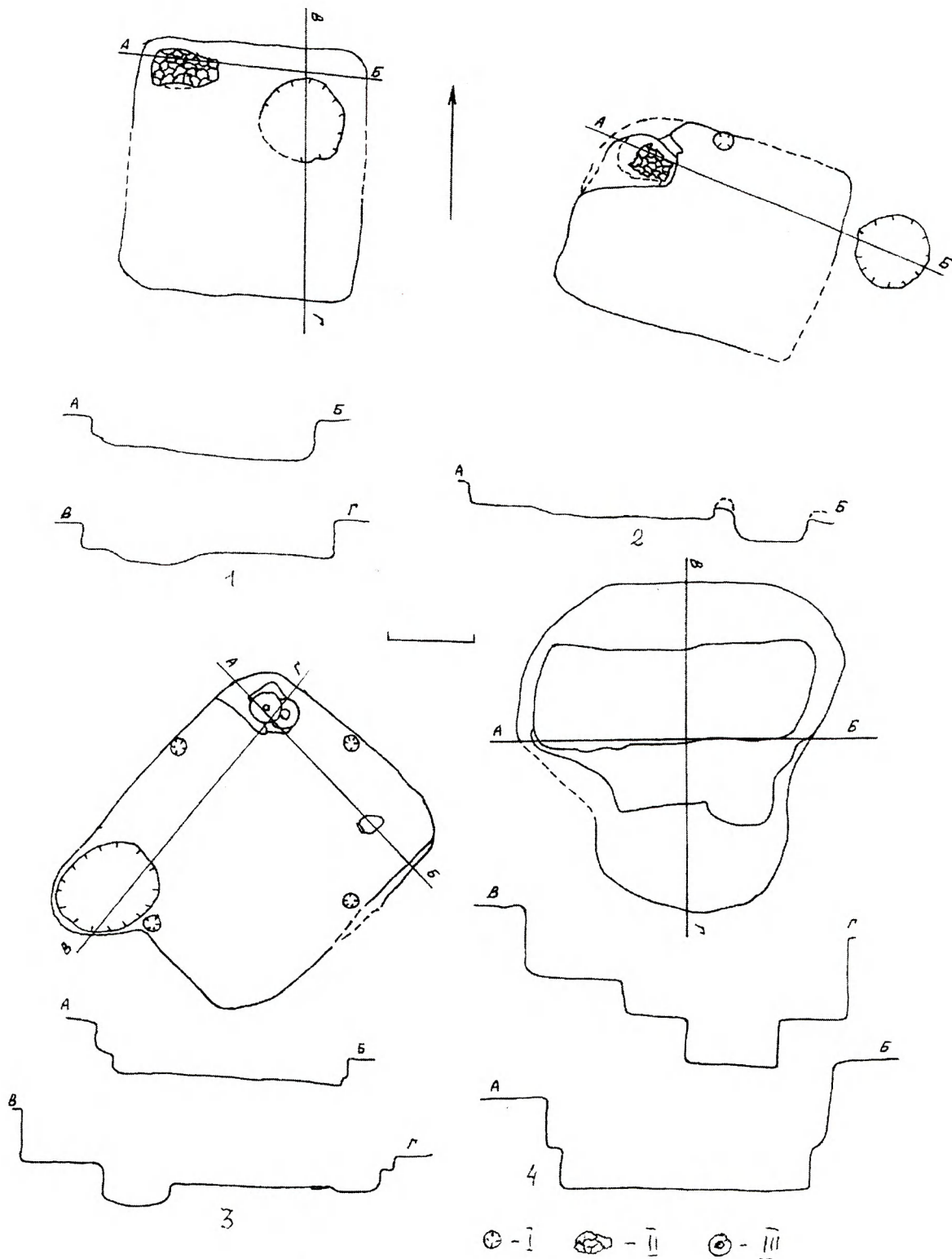
Рис. 8. Пастырське. Плани та перетини ранньосередньовічних напівземлянок № 13 (1), № 15 (2), № 16 (3) та господарської споруди (4), досліджених у середині п'ятидесятих років ХХ ст.
