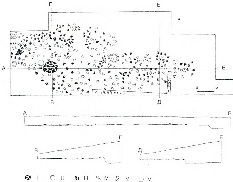
Рис. 14. Пастырське. План та перетини наземного житла скіфського часу, розкопаного у дев'яності роки XX ст.
