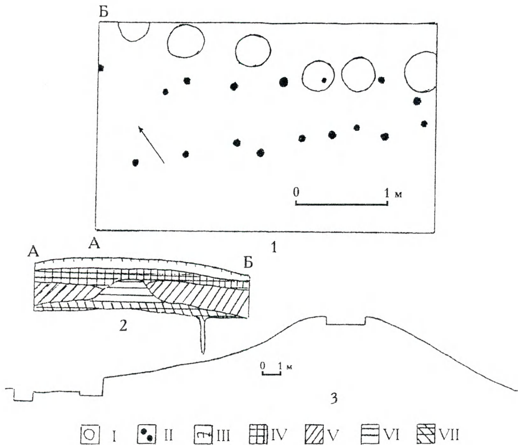
Рис. 5. Пастырське. Залишки конструкцій дослідженої частини оборонних споруд лівобережної частини городища.
