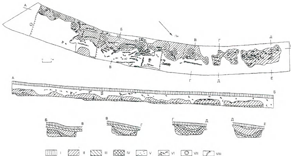
Рис. 16. Пастырське. План та перетини довгої споруди № 2.
