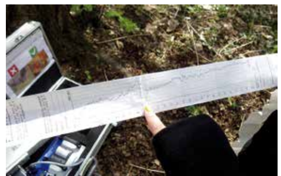
Резистограма дерева
