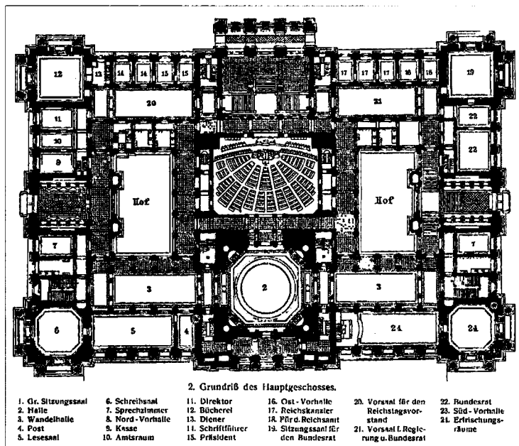
Мал. 82. План головного поверху Рейхстагу.
