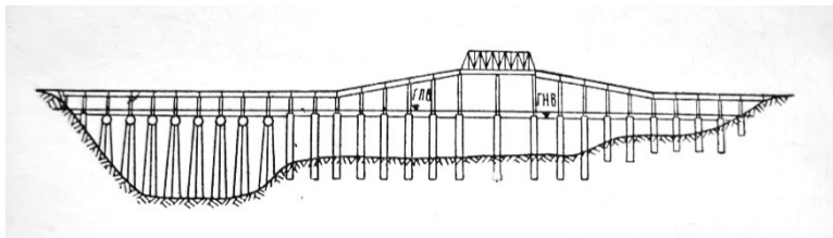
Мал.1 Схема мостового переходу з ділянкою на попливкових опорах
