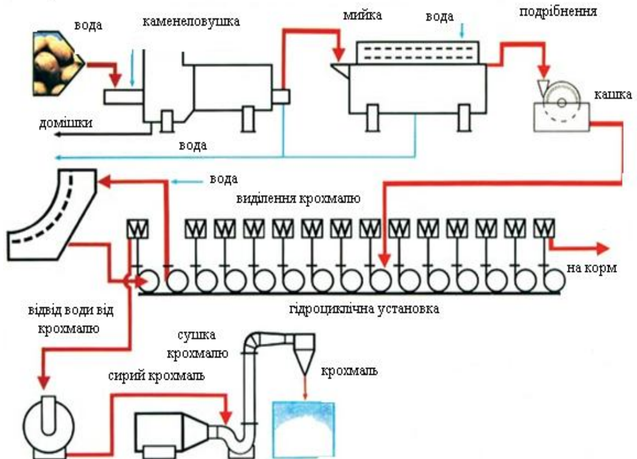
Рис. 5.4. Схема лінії переробки картоплі на крохмаль*.
