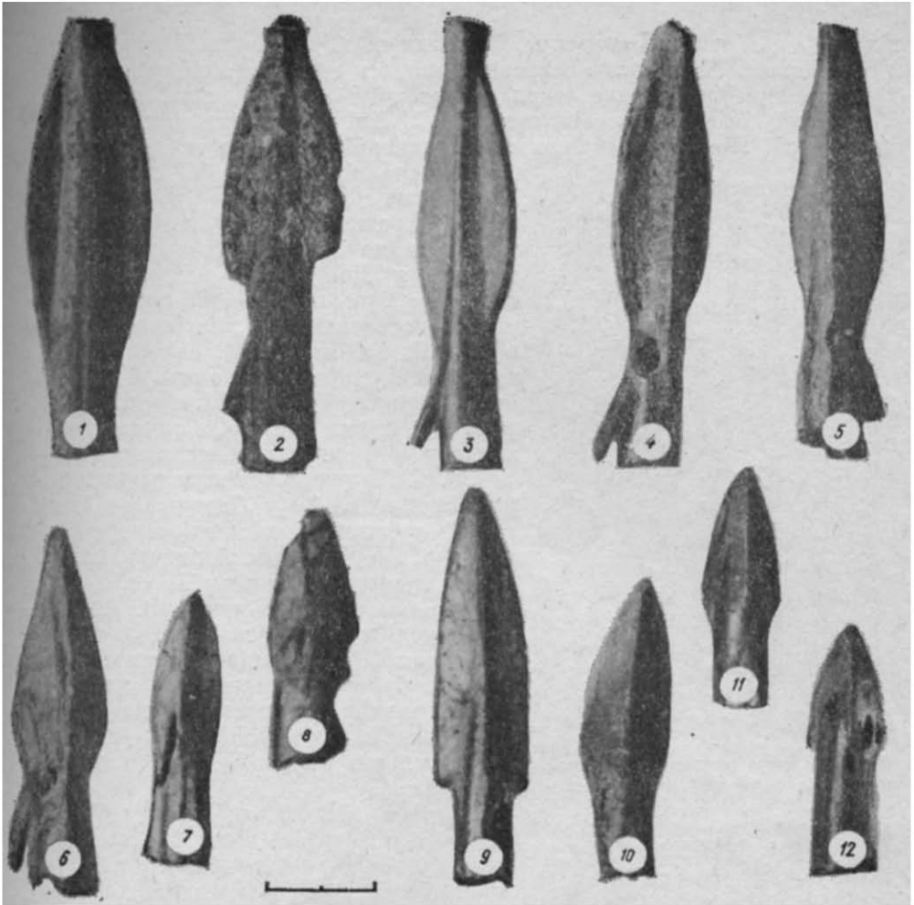
Рис. 4. Зразки бракованих наконечників стріл з Ягорлицького поселення. 1—4 — дволопатеві, 5—8 — трилопатеві, 9—12 — наконечники келерського типу.
