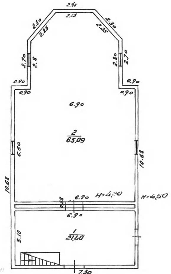
Рис. 4. План церкви с. Острів'я, 1959.
