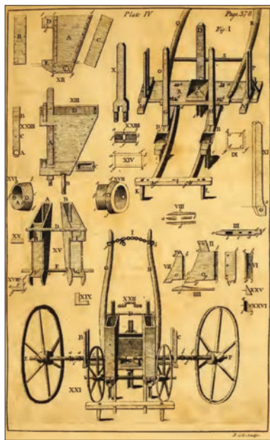
Рядкова сіялка Джетро Талла. Малюнок XVIII ст.
