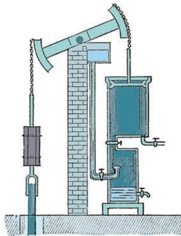
Загальна схема парового двигуна Ватта
