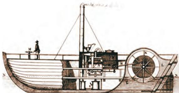
Пароплав, створений у 1801 році. Малюнок XIX ст.
