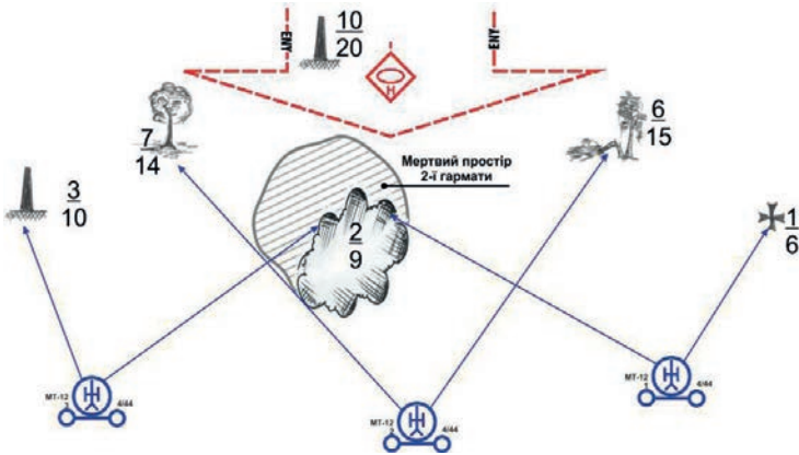
Забезпечення ураження цілей, розташованих у мертвих просторах обстрілу гармати
