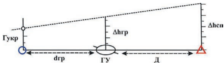
Визначення глибини укриття графічним способом
