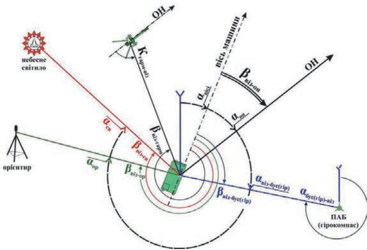
Визначення горизонтального кута \beta_{\text{виз.он}}
