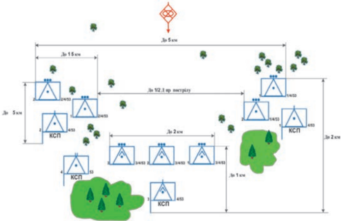
Рисунок Д5 — схема бойового порядку протитанкового резерву на рубежі розгортання (варіант).
