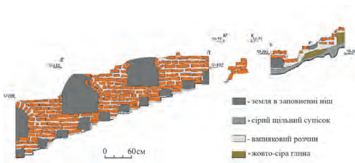
Іл. 13. План залишків цегляних конструкцій і сходинок підземного коридору та малюнок його південної стіни з нішами, розкопаних у 2019-20 рр. Комп'ютерна графіка Л. Мироненко.
