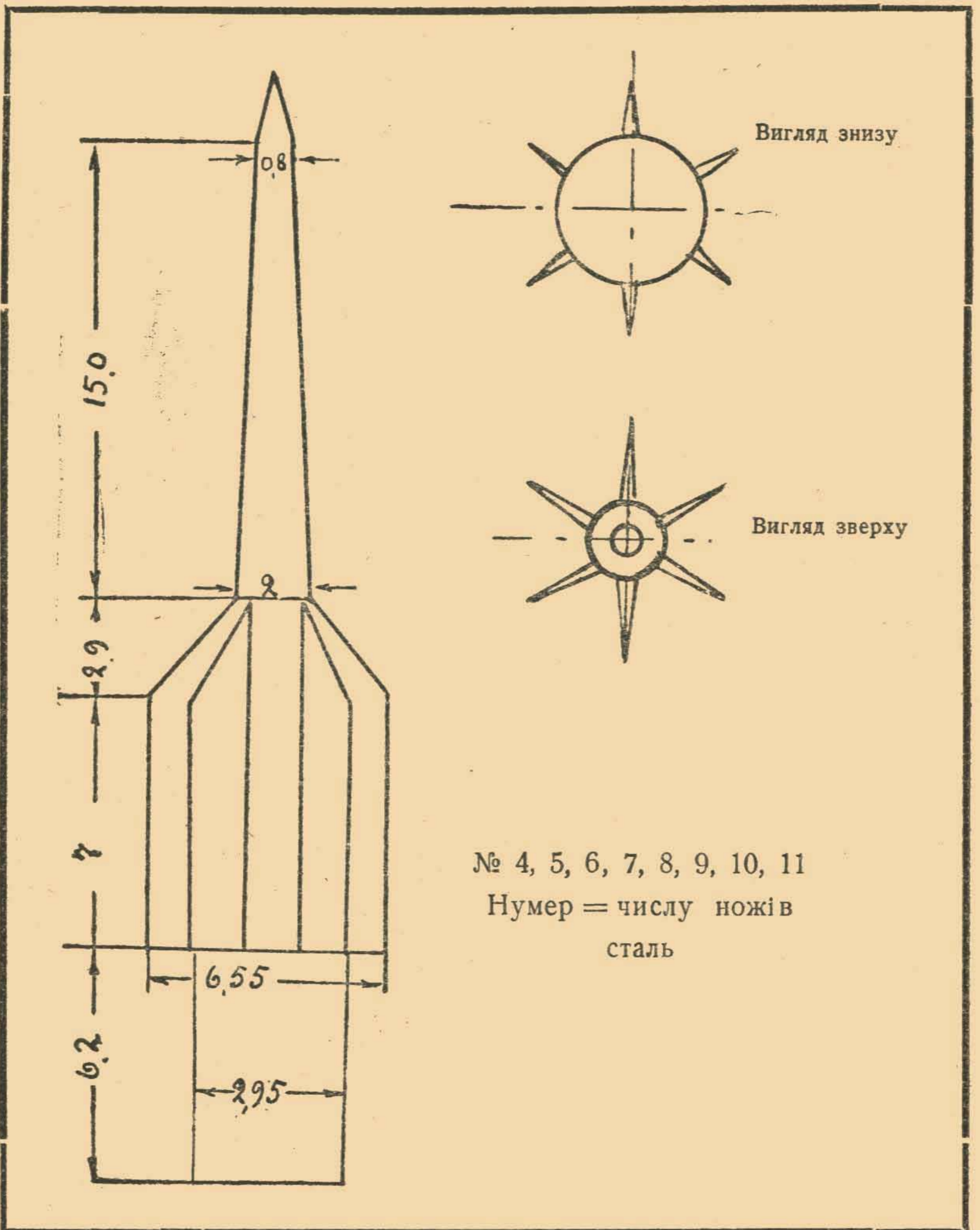
Рис. 94. Розщипник
