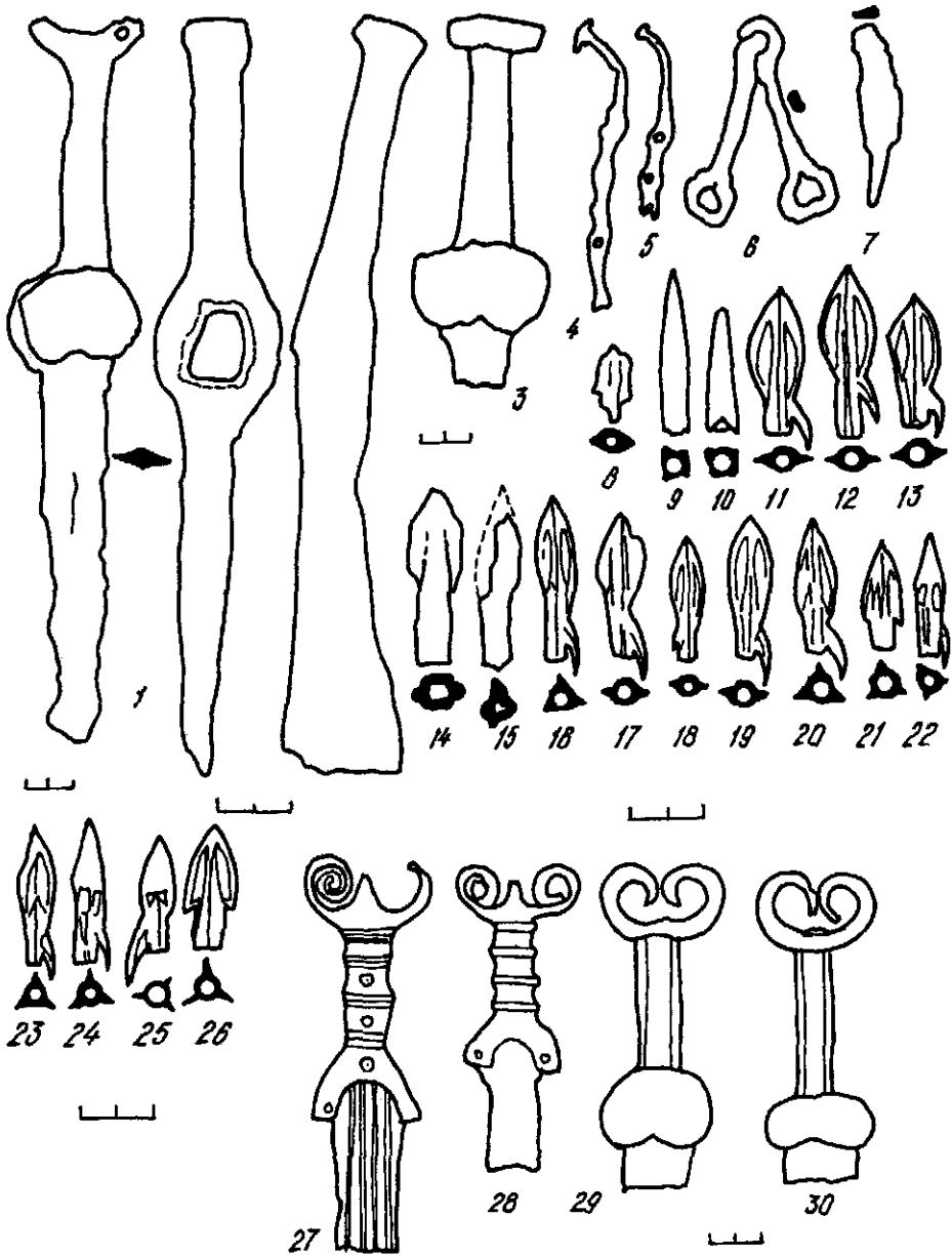
Рис. 2. Мечі та кинджали з простим антенним навершям: 1—26 — знахідки з поховання 9 могильника Кристешти (Румунія); 27 — меч типу Фермо (Північна Італія); 28 — Романд (Угорщина); 29 — Іванівський склад; 30 — Смела.
