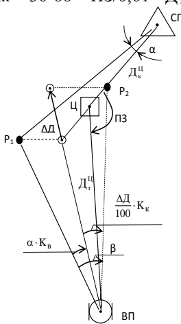
Рисунок 3.2 – Пристрілювання на себе
