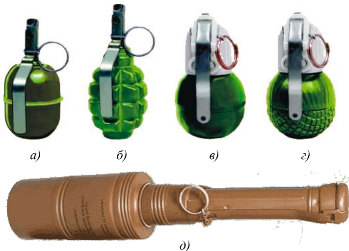
Рисунок 10.10 – Загальний вигляд ручних осколкових гранат: а) – РГД-5; б) – Ф-1; в) – РГН; г) – РГО; д) – РКГ-3
