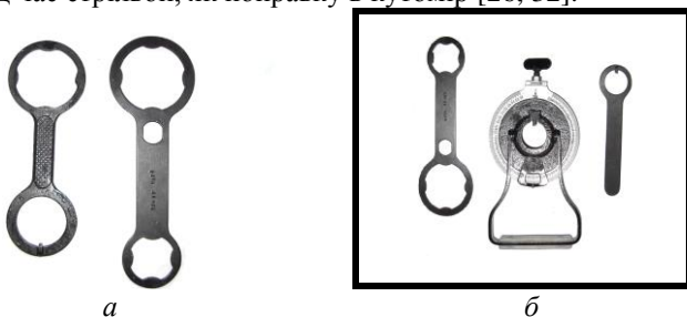
Рисунок 8.3 – Ключі для установки підричника зі складу ЗІП a – ключі для установки підричника Т-7; б – ключі для установки підричника В-90 (ключ 42-78 для згвинчування гермоковпака, та установлювального ковпачка; ключ ЗІ36; ключ ЗІ37)
