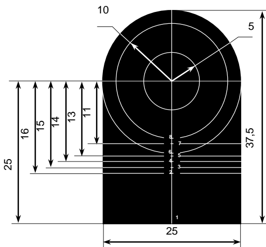
Рисунок 10.8 – Перевірочна мішень
