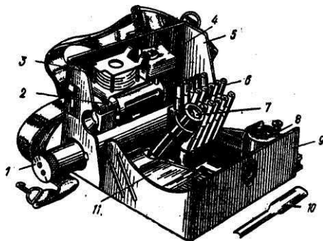
Рисунок 7.3 – Військовий прилад хімічної розвідки (ВПХР)
