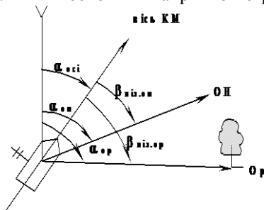
Рисунок 9.2 – Система кутів для орієнтування командирських машин
