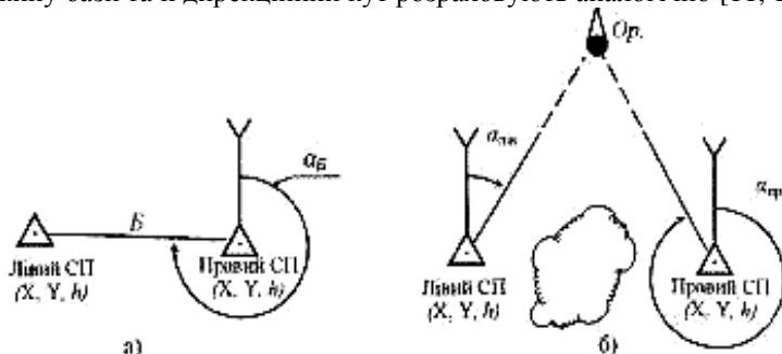
Рисунок 4.3 – Зміст топогеодезичної прив'язки пунктів спряженого спостереження:
