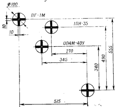
Рисунок 8.7 – Щит із перехрестями для ввірення прицільних пристроїв 100-мм ПТП МТ-12
