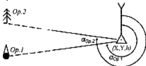
Рисунок 4.2 – Зміст топогеодезичної прив'язки спостережного пункту
