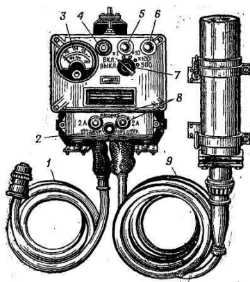
Рисунок 7.4 – Вимірювач потужності дози ДП-3Б
