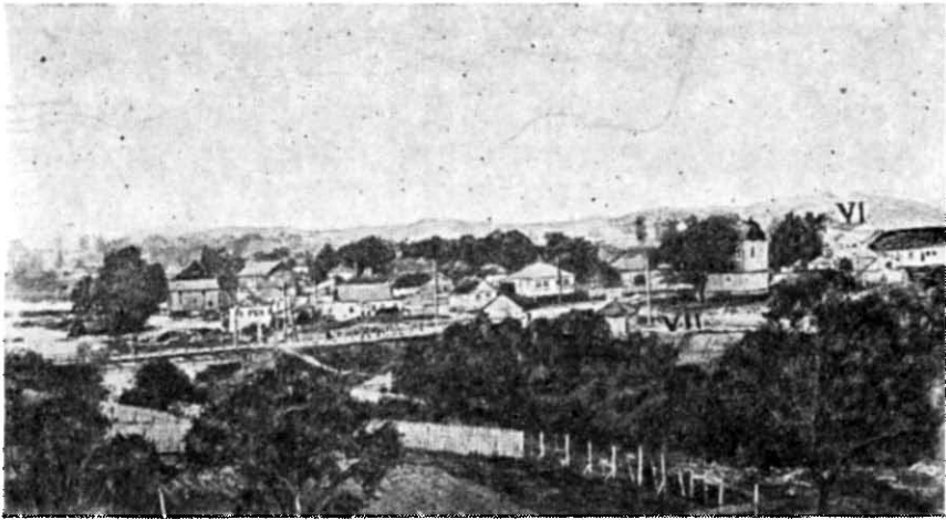
Рис. 2. м. Коростень: п. VII — місце, де знаходиться стоянка, відкрита В. В. Хвойком; п. VI — місцезнаходження кремінних знарядь.
