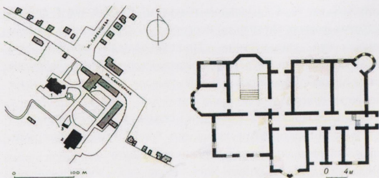
План садиби і першого поверху головної будівлі
