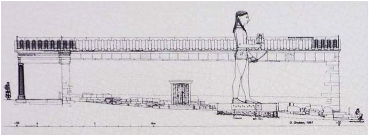
Fig. 44. — L'Oikos des Naxiens : perspective et coupe restituées de l'Ouest.
