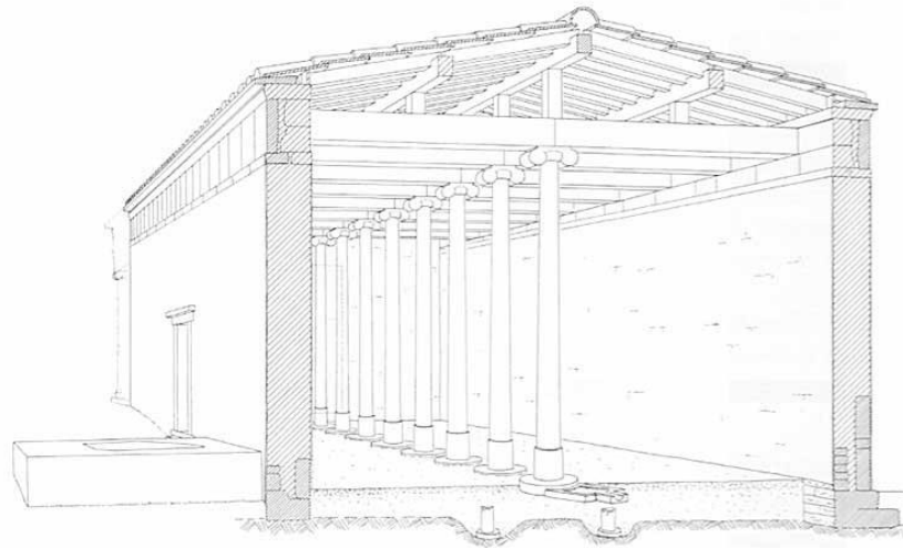
Fig. 44. — L'Oikos des Naxiens : perspective et coupe restituées de l'Ouest.
