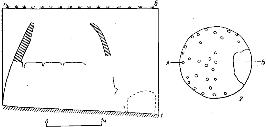
Рис. 3. Гончарне горно. Розріз (1) і план перегородки з люфтами (2).
